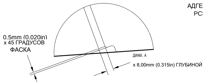
ДЕТАЛЬ Y (БЕЗ СМАЗОЧНОГО АДАПТЕРА)
