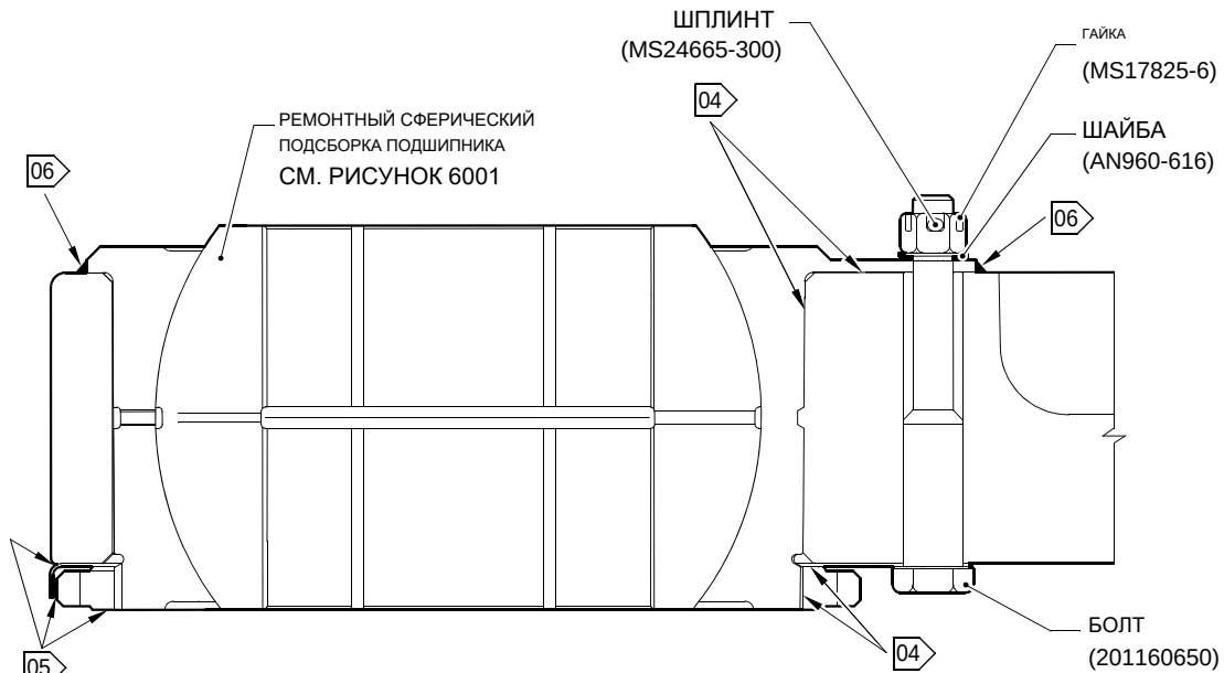
СЕЧЕНИЕ Z-Z
