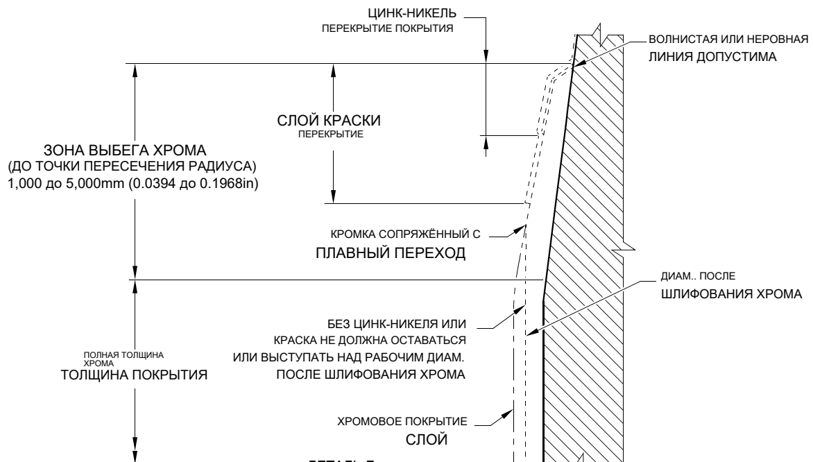
ЗАВЕРШЕНИЕ ХРОМИРОВАНИЯ ПОЯСКОВ А,В,С (ТИПОВО)
