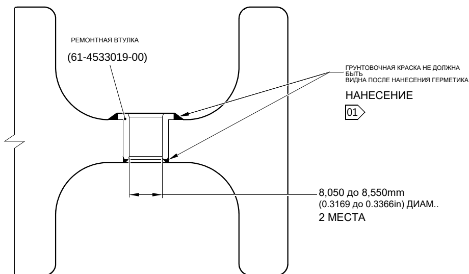
СЕЧЕНИЕ Y-Y (С ВЕРХНИМ)
