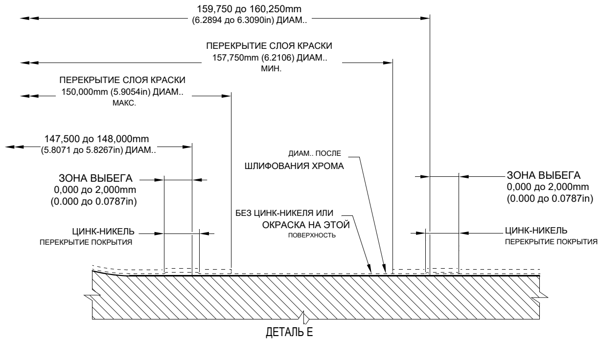
ЗАВЕРШЕНИЕ ХРОМИРОВАНИЯ ТОРЦА ТОРМОЗНОГО ФЛАНЦА (ТИПОВО)
