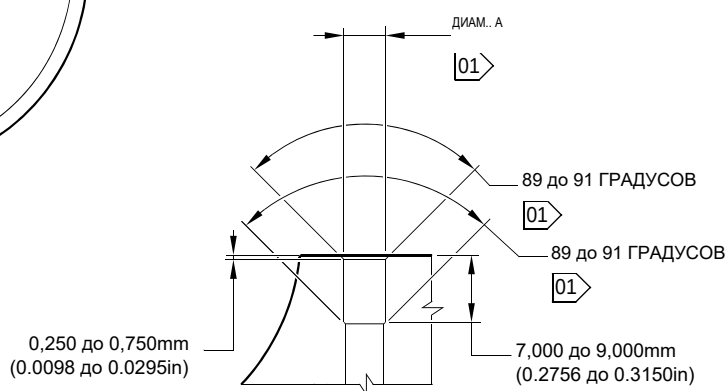
ДЕТАЛЬ С
