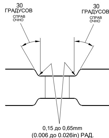
ДЕТАЛЬ E
