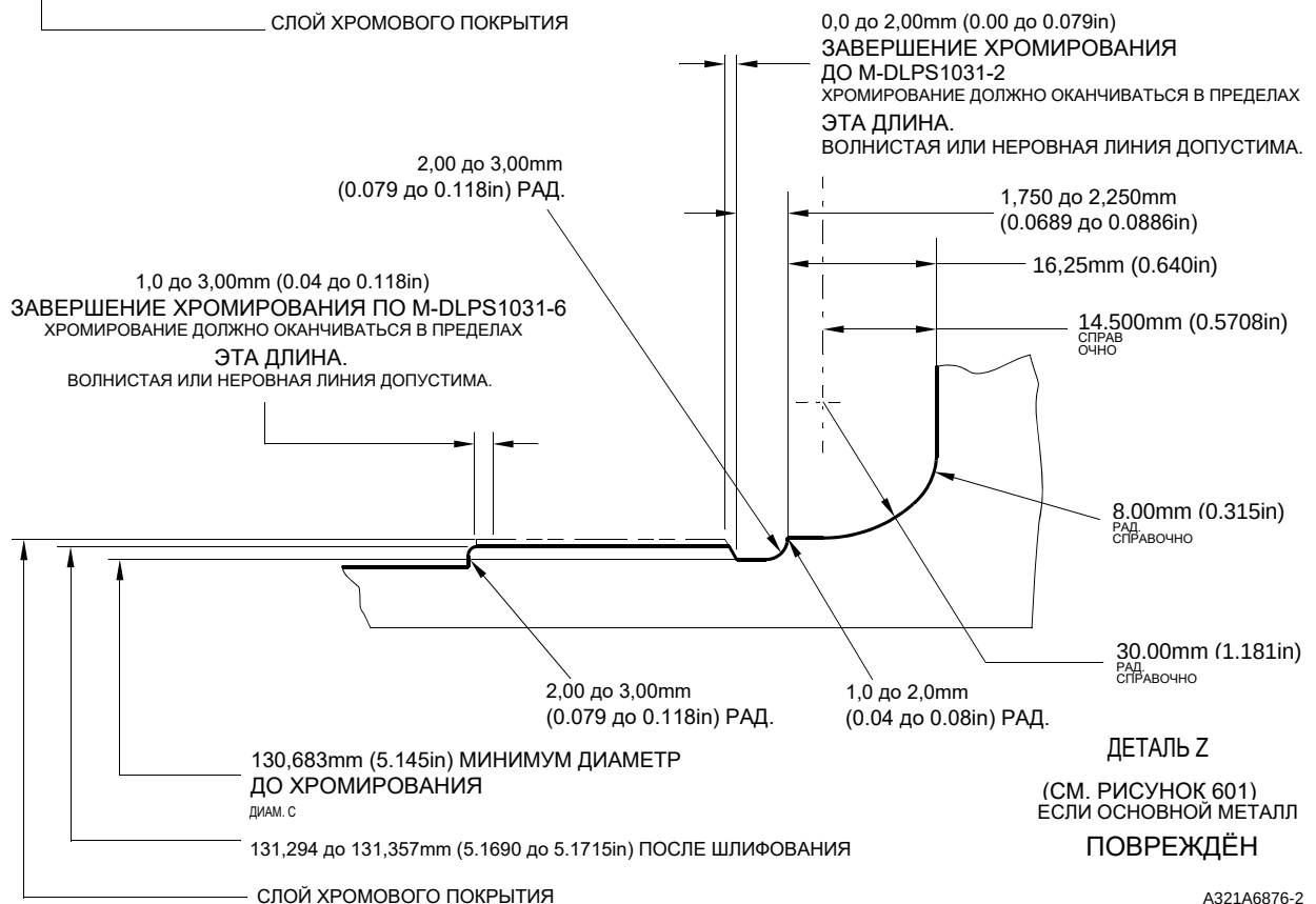
Ремонт скользящей трубы Рисунок 602
