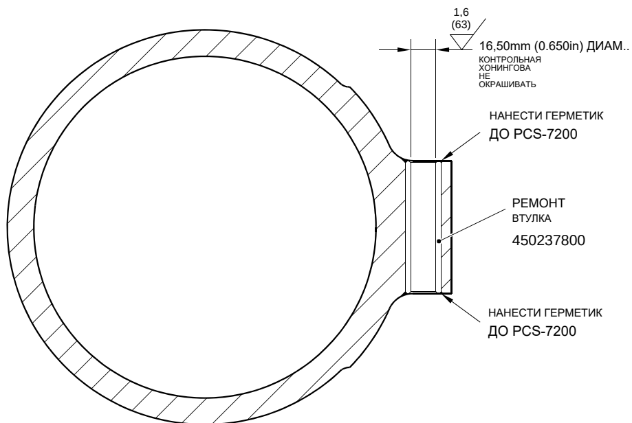
СЕЧЕНИЕ Z-Z
