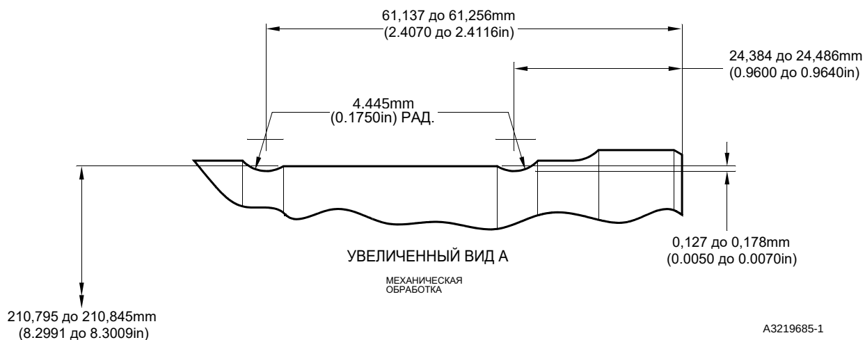
Ремонт под сборки нижнего подшипника Рисунок 601
