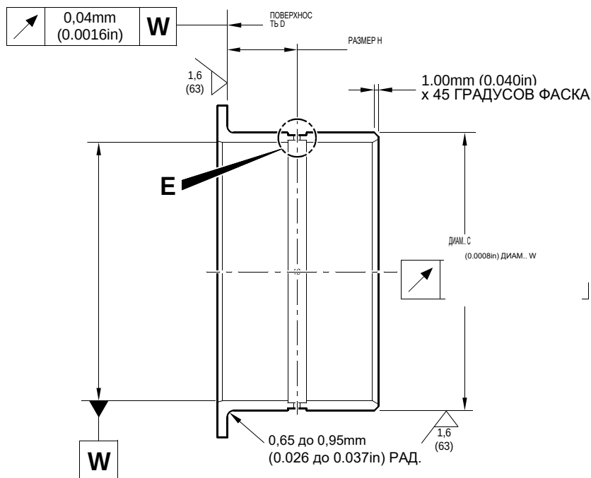
РЕМОНТНАЯ ВТУЛКА
