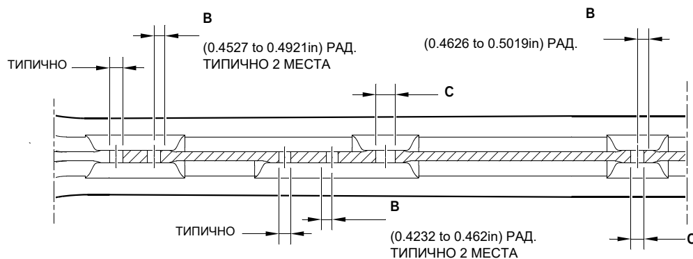
СЕЧЕНИЕ В-В ОТВЕРСТИЯ ПОДКОСА ТОЛЬКО ДЛЯ КОРПУСА СТОЙКИ (20-410С, 20-420С)
