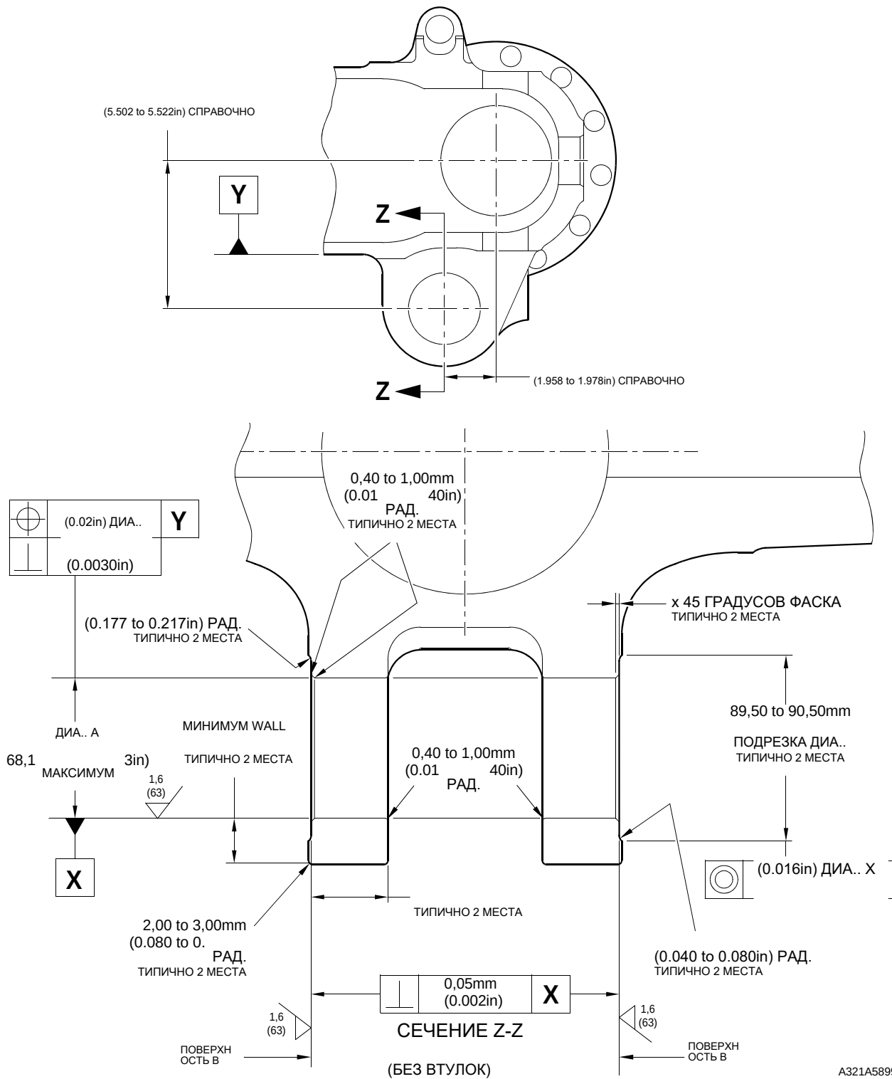
Ремонт скользящей трубы – мехобработка Рисунок 601
