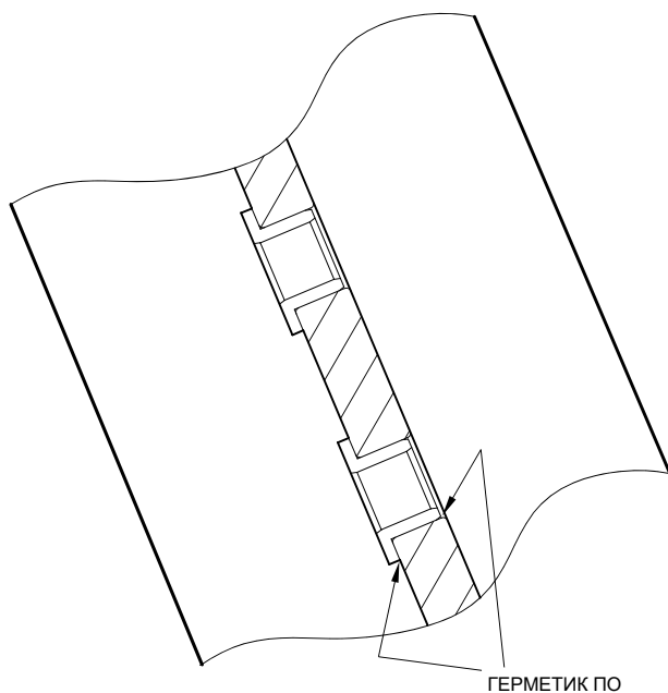
РАД СЕЧЕНИЕ Z-Z С РЕМОНТНЫМИ ВТУЛКАМИ
