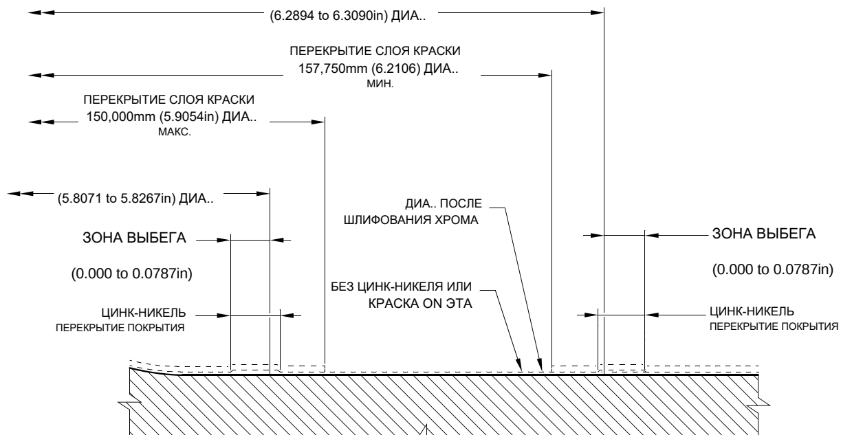
ДЕТАЛЬ Е
