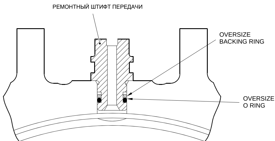
ТИПИЧНО INSTALLATION OF РЕМОНТНЫЕ КОМПОНЕНТЫ
