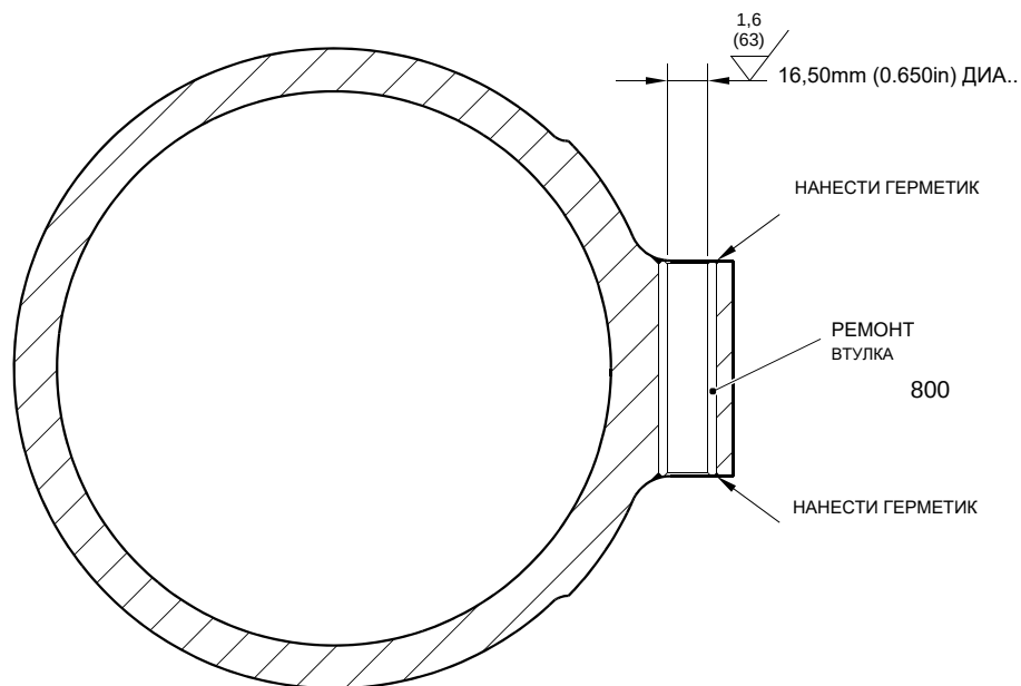
СЕЧЕНИЕ Z-Z
