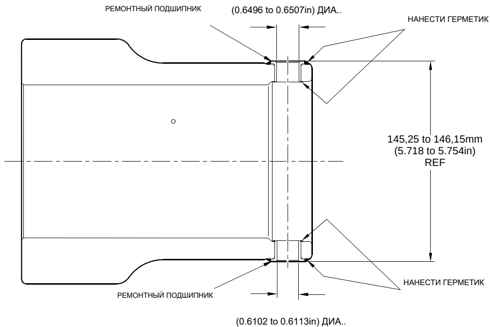
СЕЧЕНИЕ Z-Z (СМ. РИСУНОК 601)
