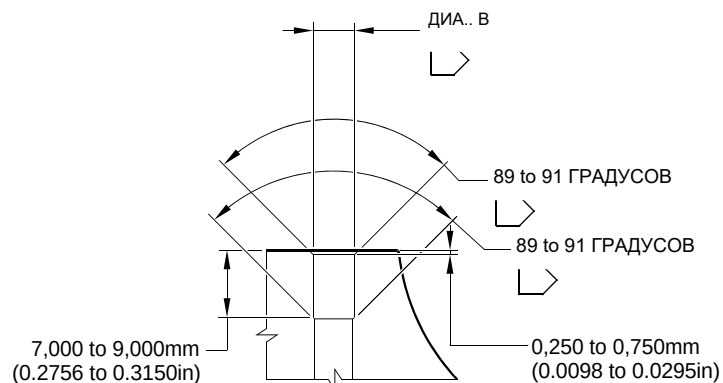
ДЕТАЛЬ В
