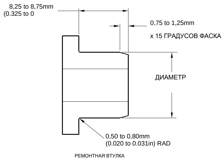
РЕМОНТНАЯ ВТУЛКА
