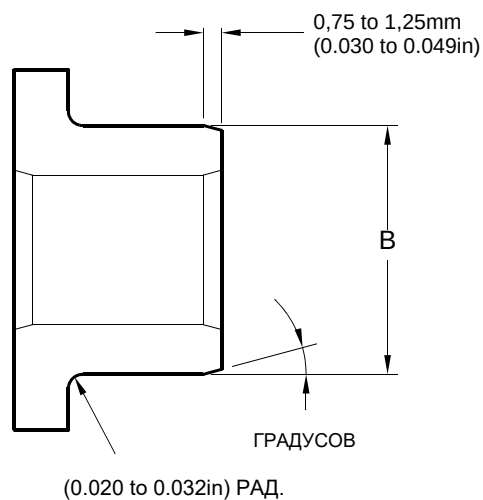
РЕМОНТНАЯ ВТУЛКА 450237819
