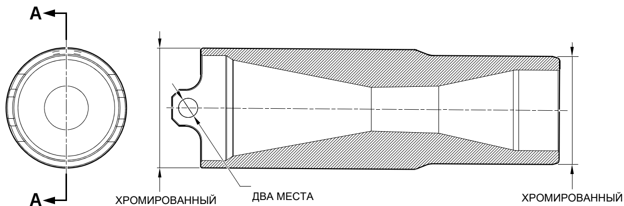
СЕЧЕНИЕ А-А
