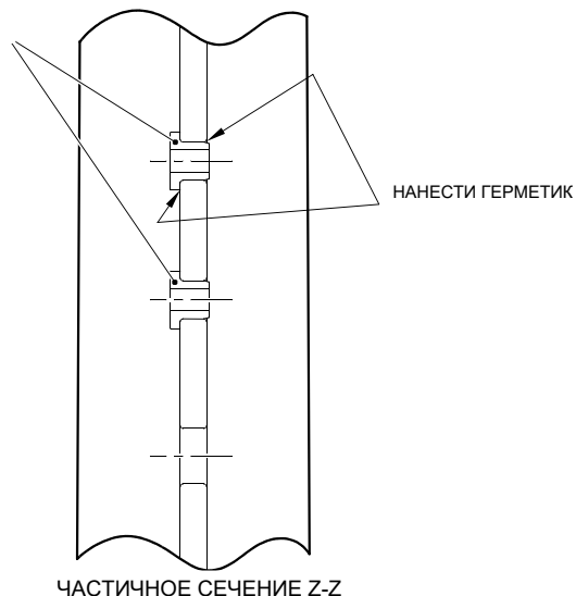
ЧАСТИЧНОЕ СЕЧЕНИЕ Z-Z СМ. РИСУНОК 601 (С РЕМОНТНЫМИ ВТУЛКАМИ)
