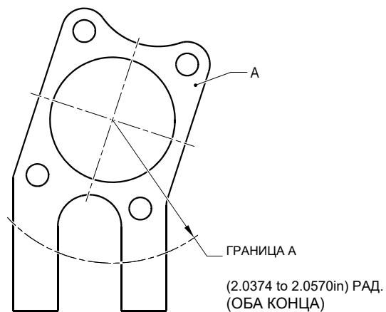
ВИД А
