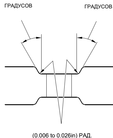
ДЕТАЛЬ Е ТYP. 4 МЕСТА
