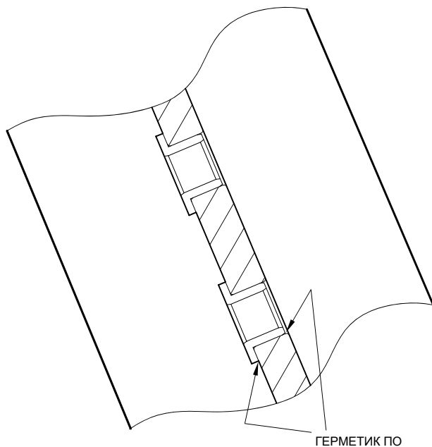
ЧАСТИЧНОЕ СЕЧЕНИЕ Z-Z С РЕМОНТНЫМИ ВТУЛКАМИ
