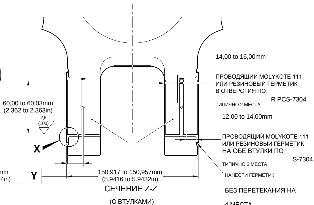
Ремонтные втулки – мехобработка и установка Рисунок 602
