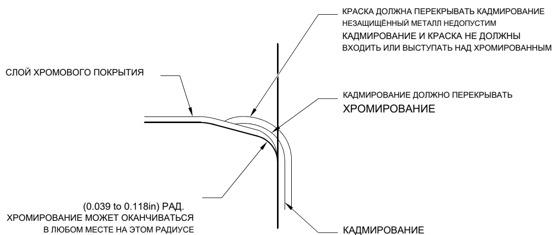
ДЕТАЛЬ W
