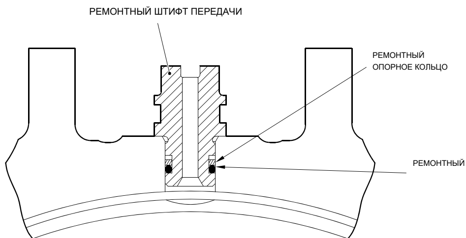
ТИПИЧНО УСТАНОВКА OF РЕМОНТНЫЕ КОМПОНЕНТЫ
