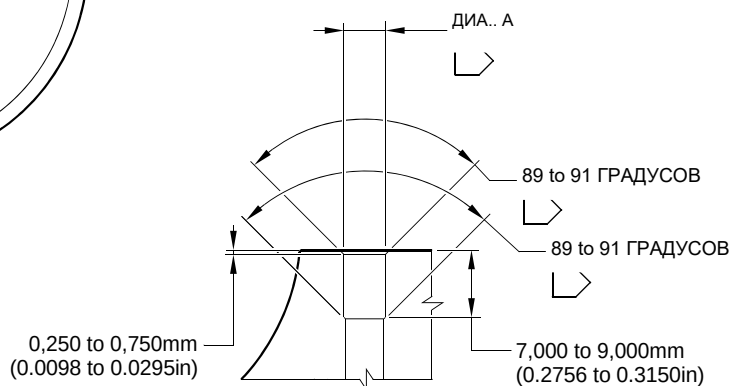
ДЕТАЛЬ С
