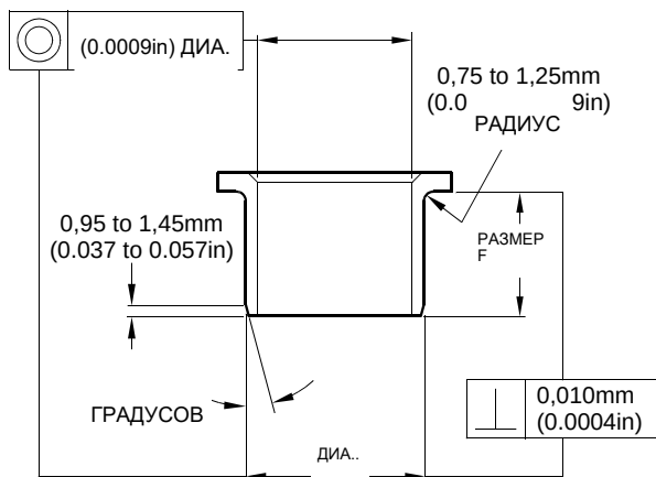
РЕМОНТНЫЙ ПОДШИПНИК
