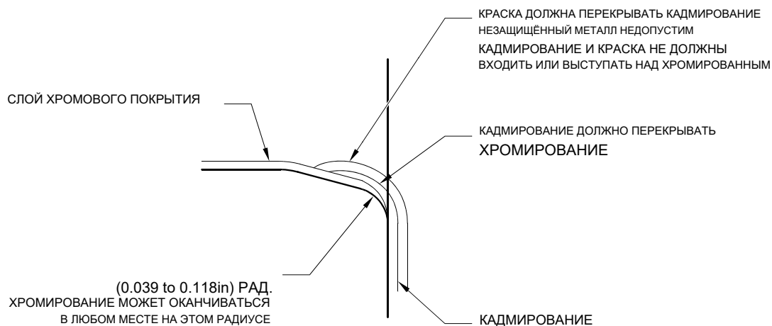
ДЕТАЛЬ W
