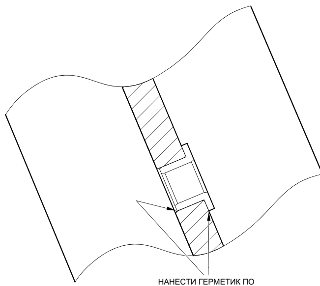
СЕЧЕНИЕ Z-Z С ВТУЛКА
