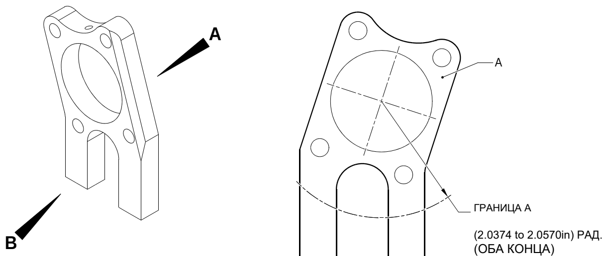
ВИД А
