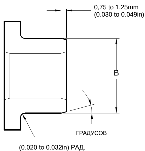
РЕМОНТНАЯ ВТУЛКА 450237819
