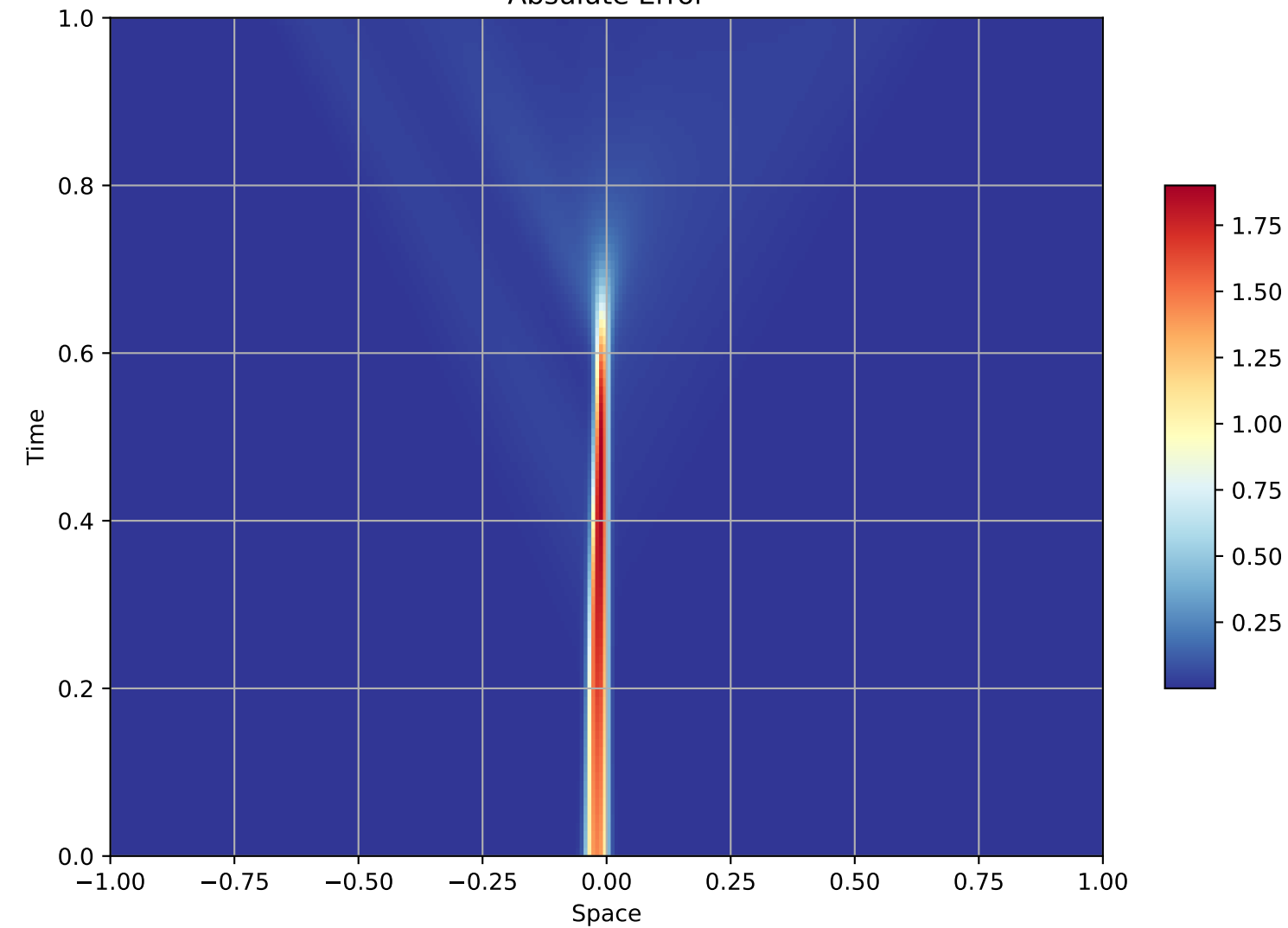
Absolute Error
