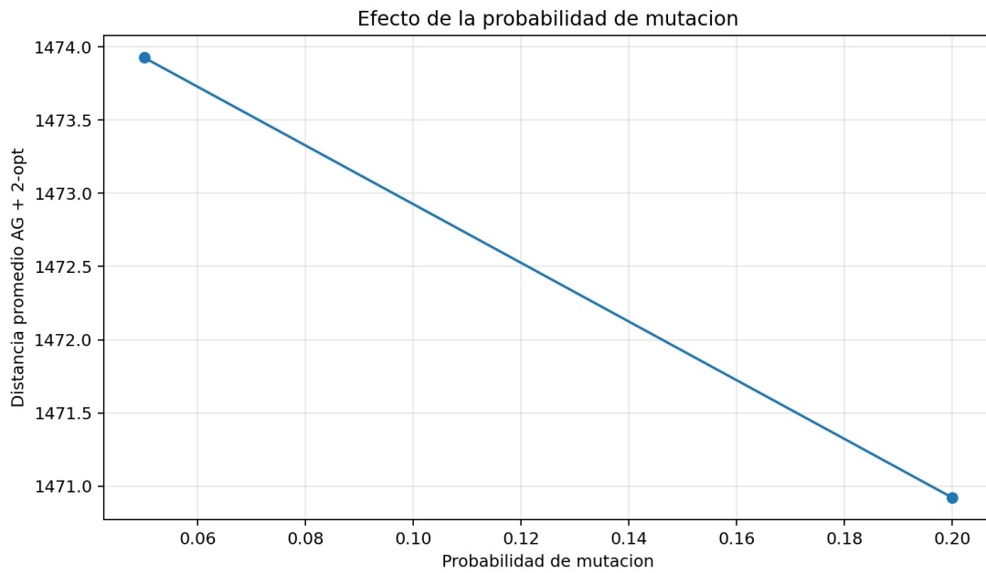
Figura 8. Efecto de la probabilidad de mutación en la distancia promedio.
