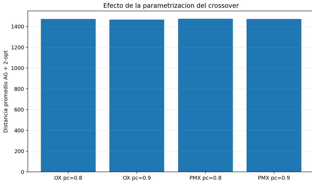
Figura 9. Efecto del tipo y probabilidad de crossover.
