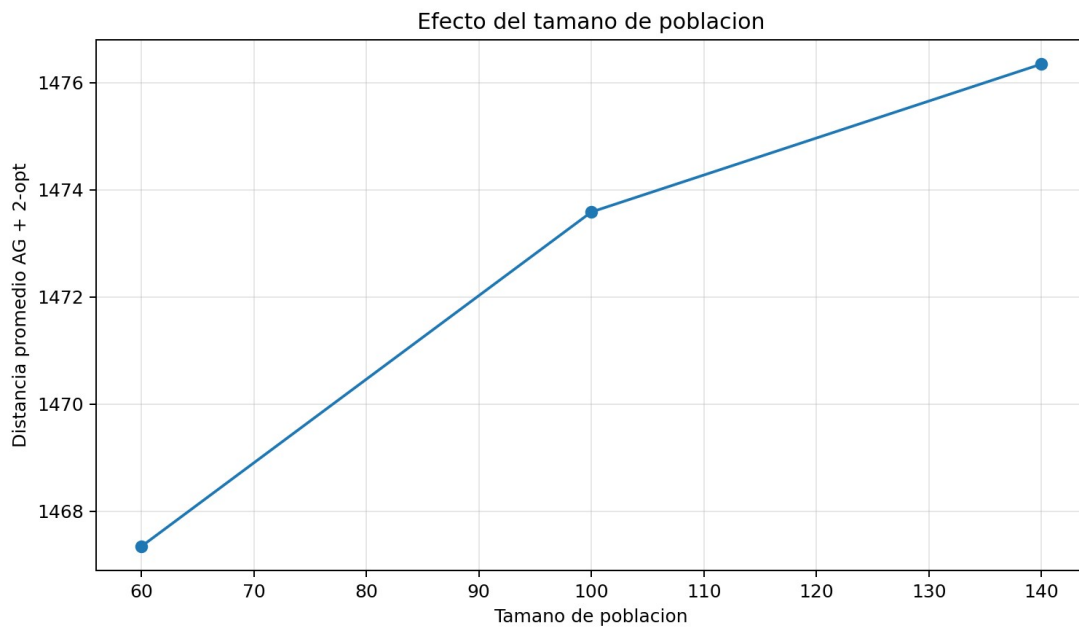
Figura 7. Efecto del tamaño de población en la distancia promedio.
