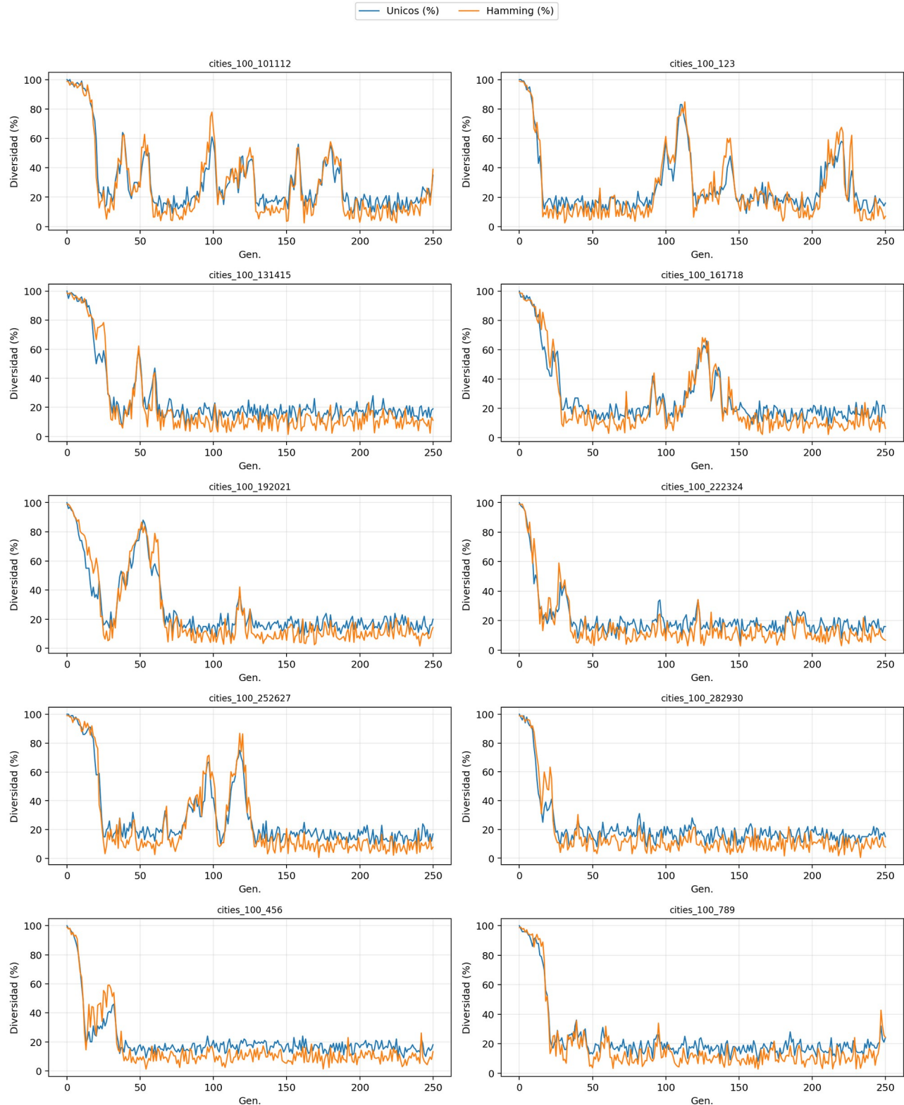
Figura 3. Evolucion de diversidad poblacional por dataset.
