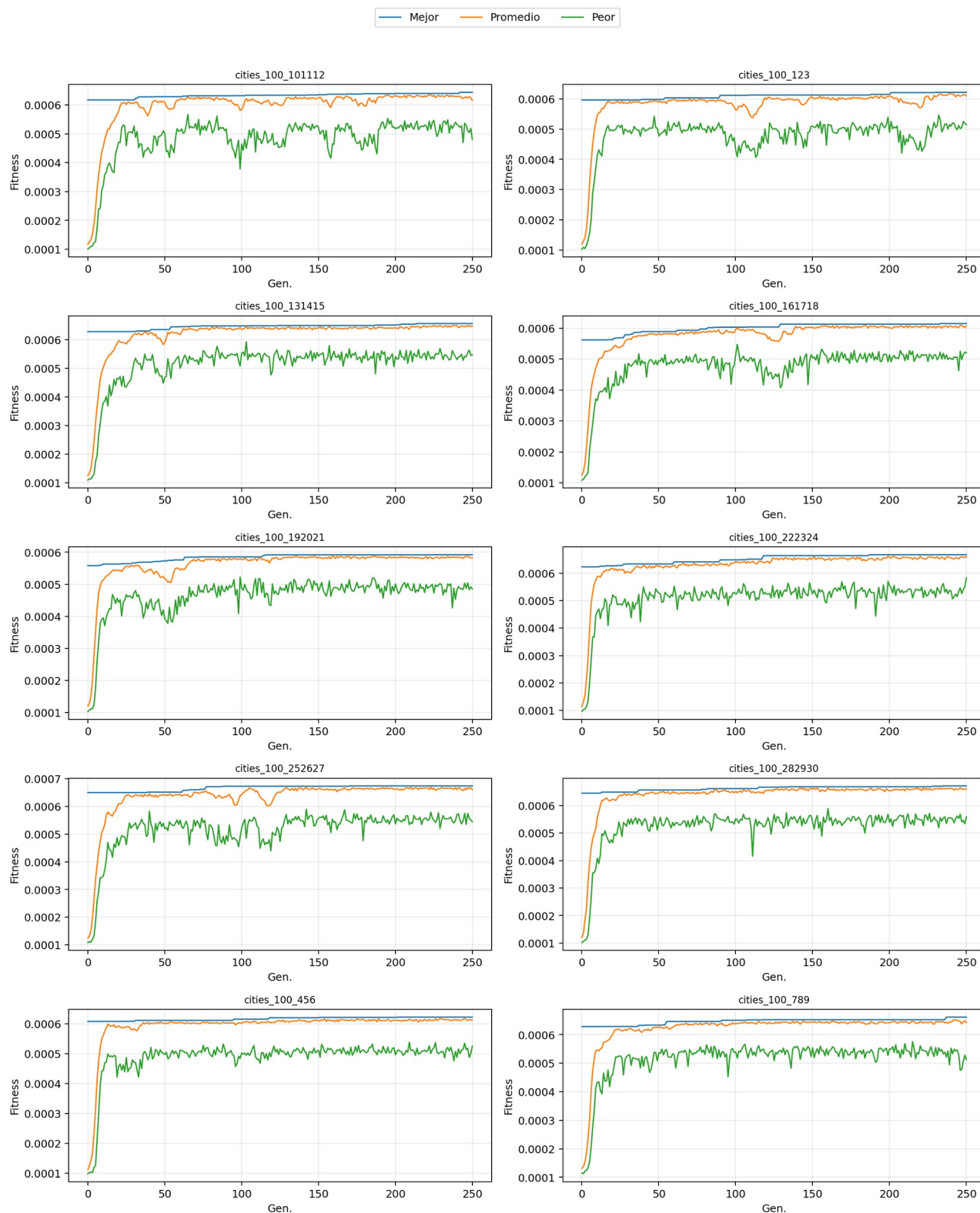
Figura 1. Evolucion del mejor fitness, fitness promedio y peor fitness por dataset.
