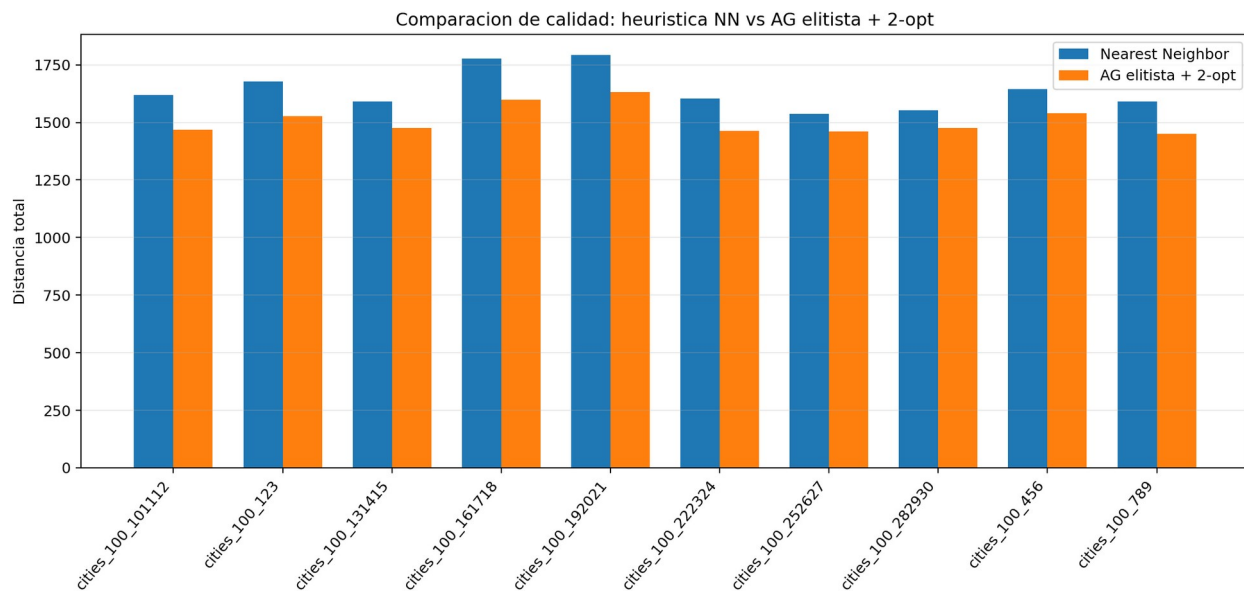
Figura 2. Comparacion de distancia final entre Nearest Neighbor y AG elitista + 2-opt.
