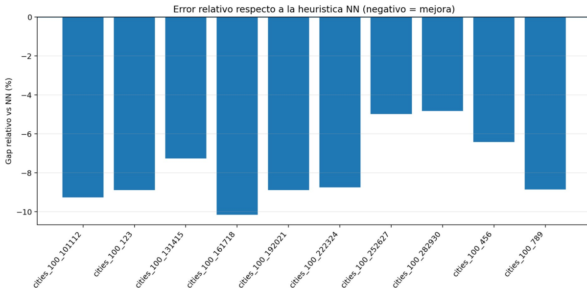
Figura 5. Gap relativo frente a Nearest Neighbor. Valores negativos representan mejora.
