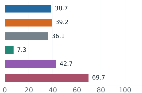
TriviaQA (%) ↑
