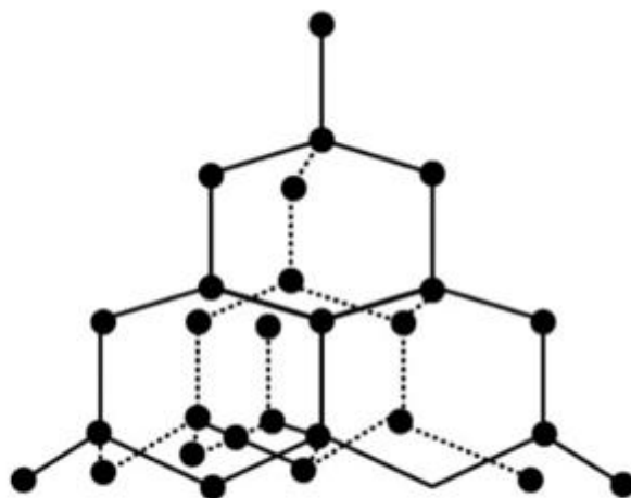
金刚石结构
