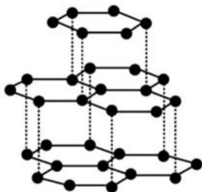
石墨结构
