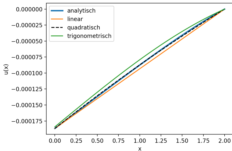
Abbildung 1: Verschiebung u(x) : analytisch vs. Näherungen (linear, quadratisch, trigonometrisch).
