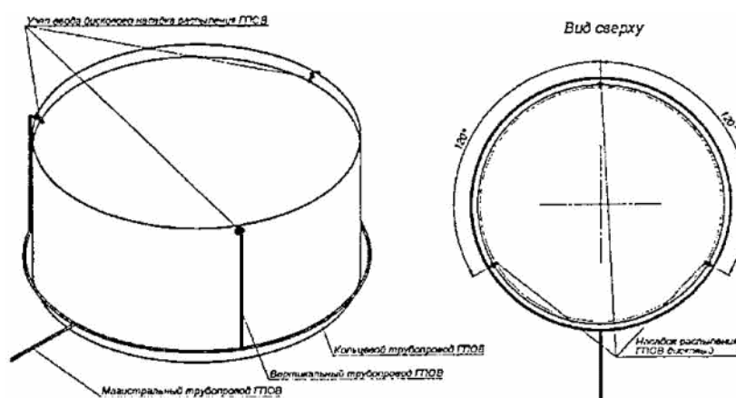
Рисунок В.1 - Схема расположения насадков распыления ГПОВ
