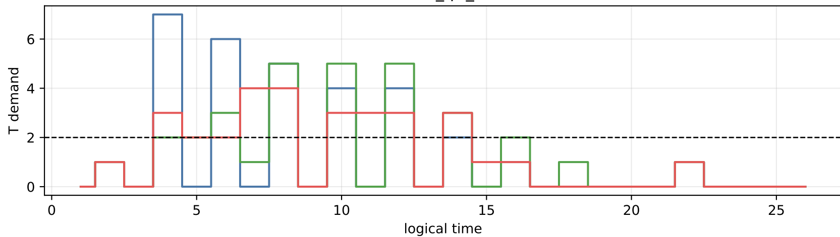
exact_qft_n8
