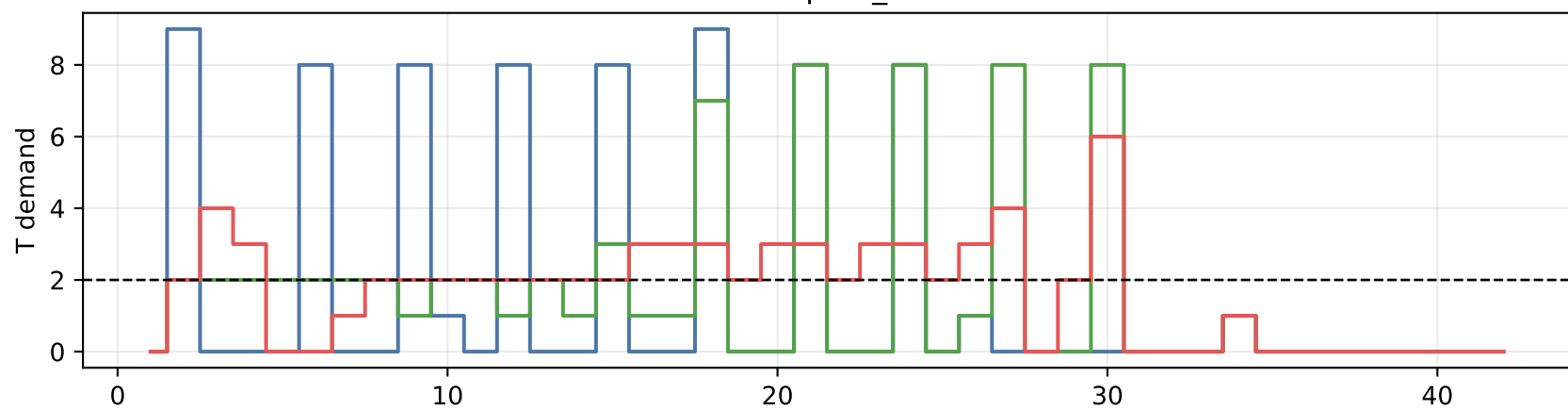
exact_qft_n8
