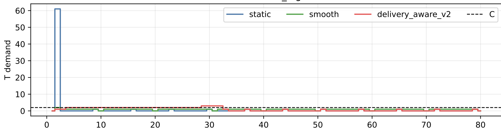
multiplier_n8
