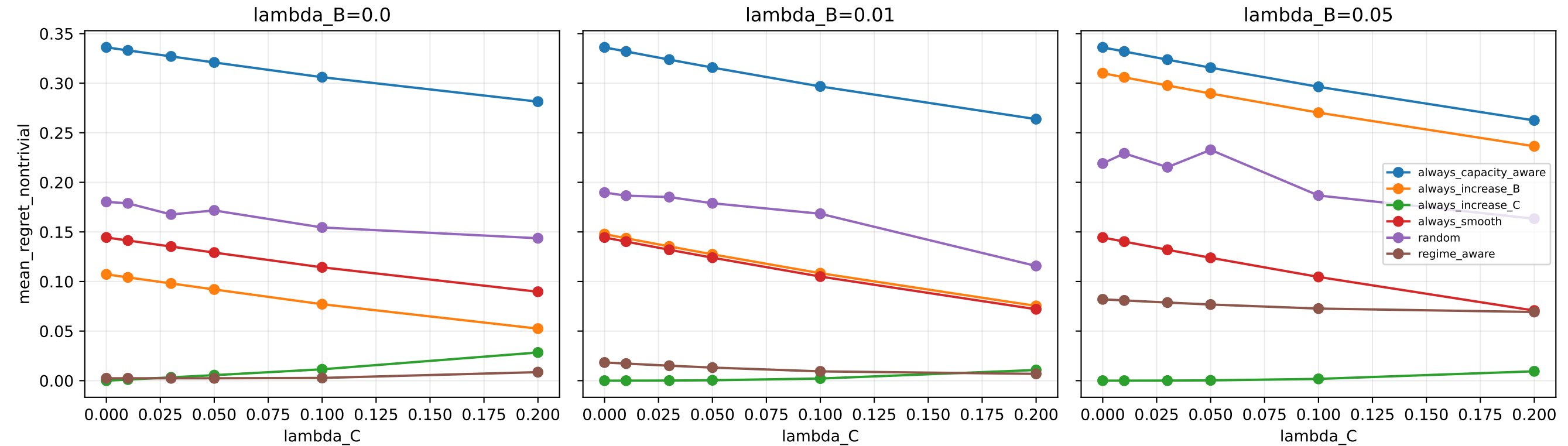
Nontrivial mean regret
