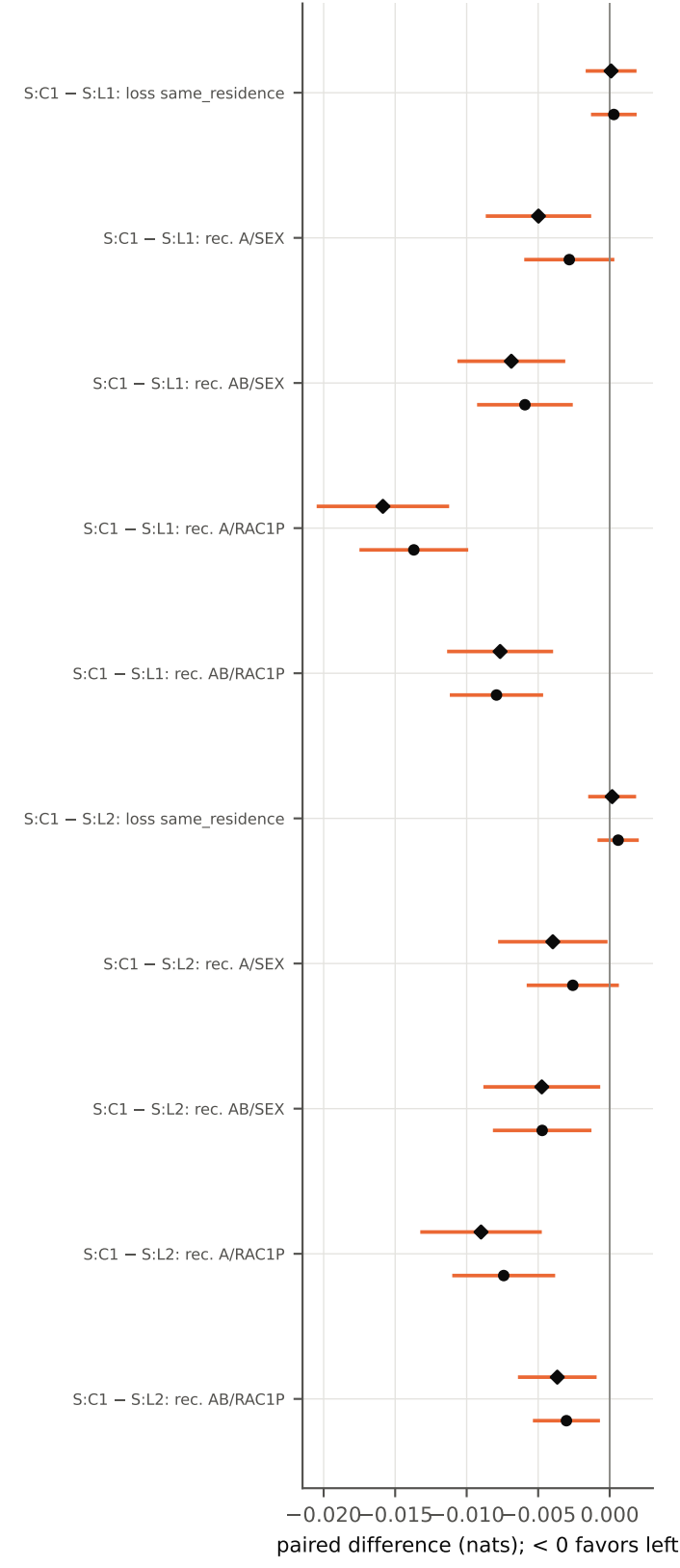
F1 primary (c = 2.93)
