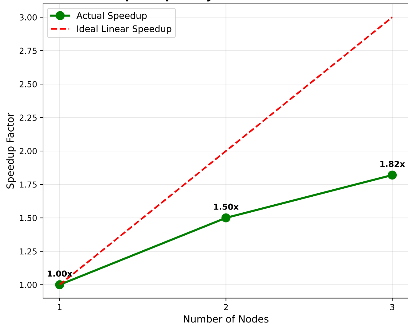
Speedup Analysis: Actual vs Ideal
