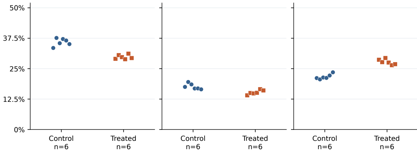
Type D
