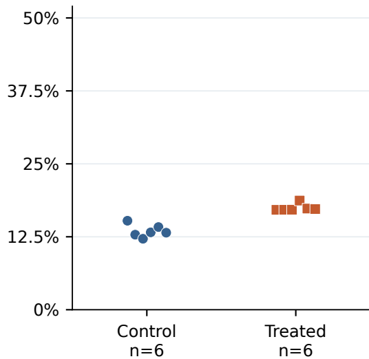
Type D
