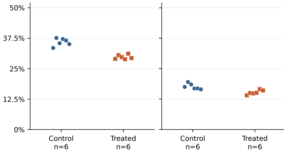
Type D
