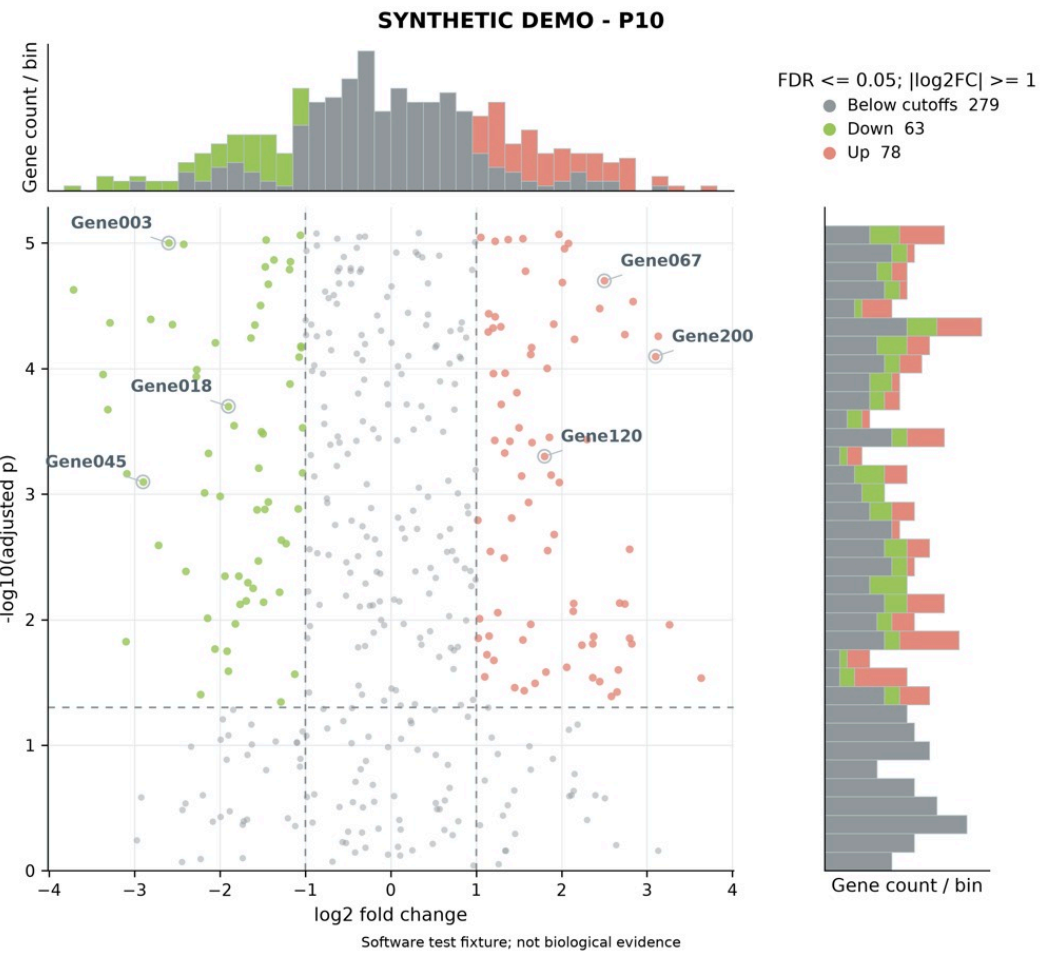
P 1 0 / P 1 0 火山图+上下／侧面堆积分布 · 默认形式
