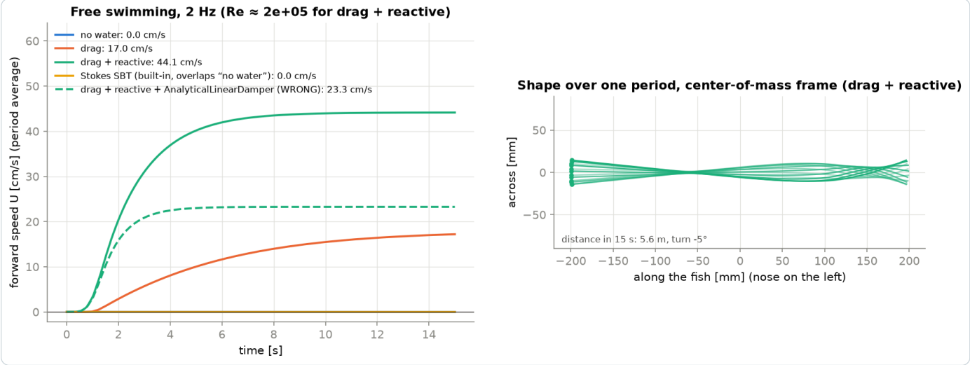
Etap 4: wybór modelu wody decyduje o wyniku. Bez siły reakcyjnej (Lighthilla) ryba osiąga 17 cm/s; model Stokesa daje zero.
