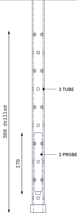
DETAIL A: PROBE ZONE
