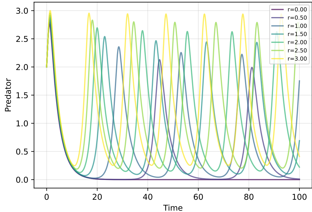
Predator — r sweep
