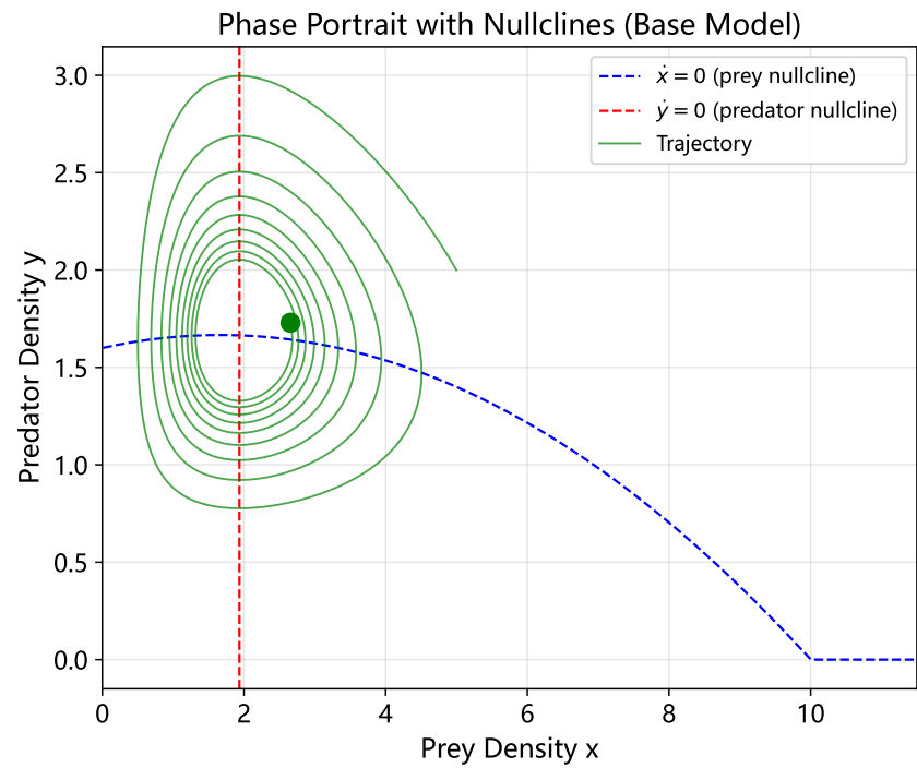
图 10: 基础模型的零斜率线与相轨迹
