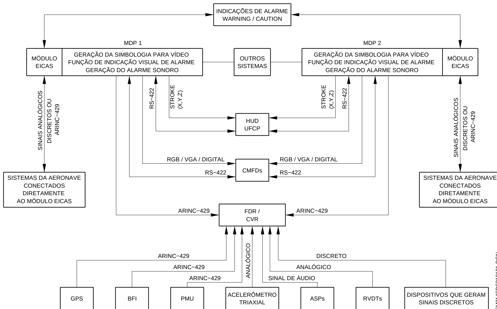
SISTEMAS DE INDICAÇÃO E REGISTRO - DIAGRAMA DE BLOCOS, Folha 1
