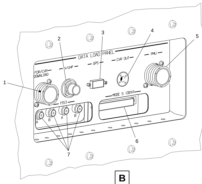
PAINEL DATA LOAD - LOCALIZAÇÃO, Folha 1
