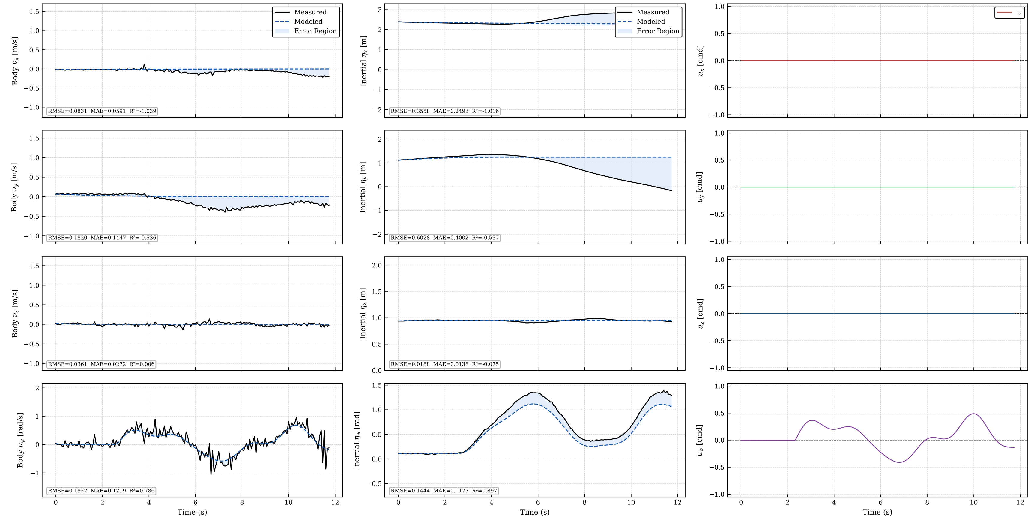
Validation — uncoupled_sine_udPsidot_08_Aug_2026_17h09min_B10_15Hz_COMPLETEO.csv
