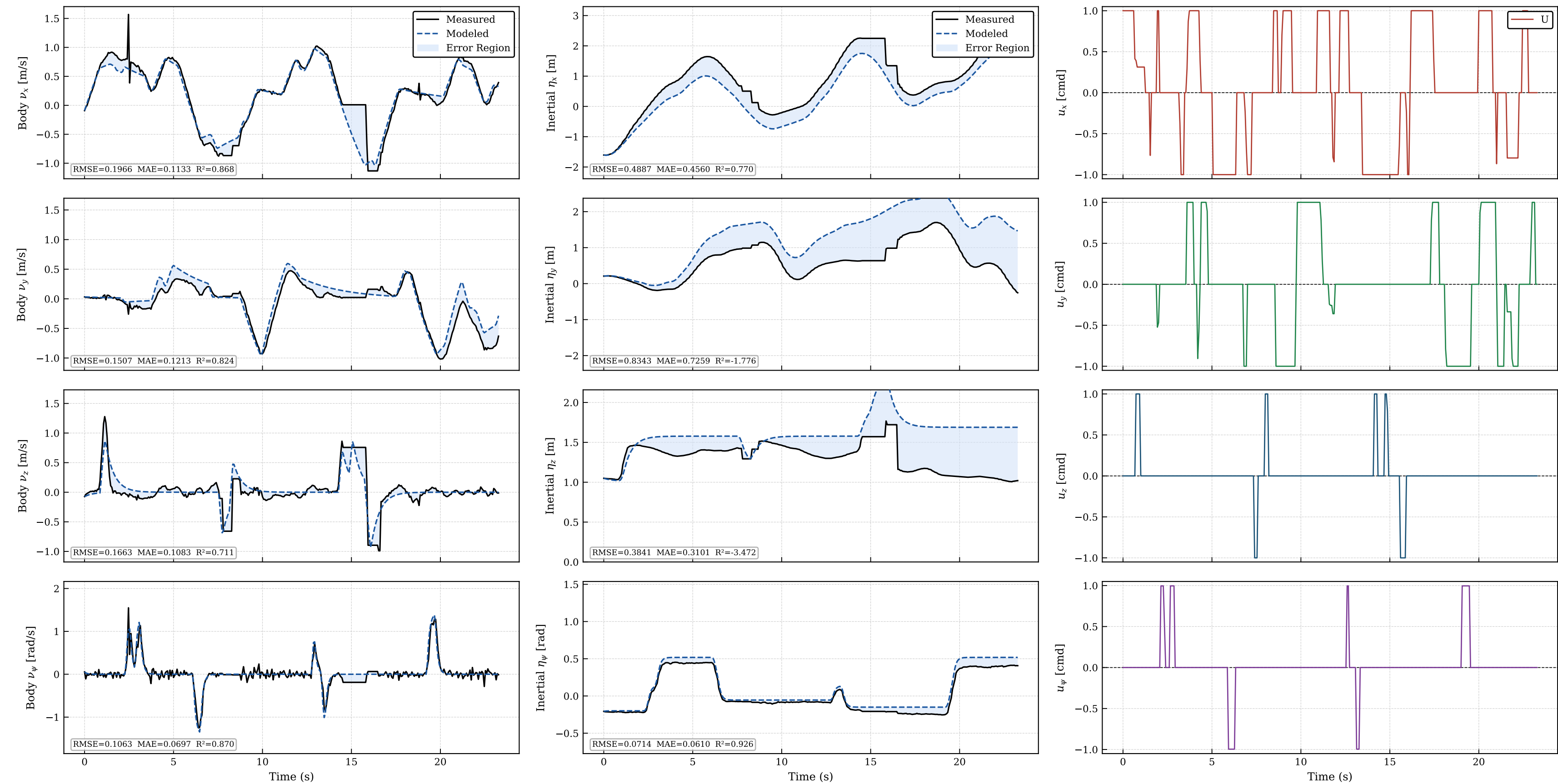
Validation — coupled_sine_joystick_09_Aug_2026_11h44min_B10_15Hz_COMPLETO.csv
