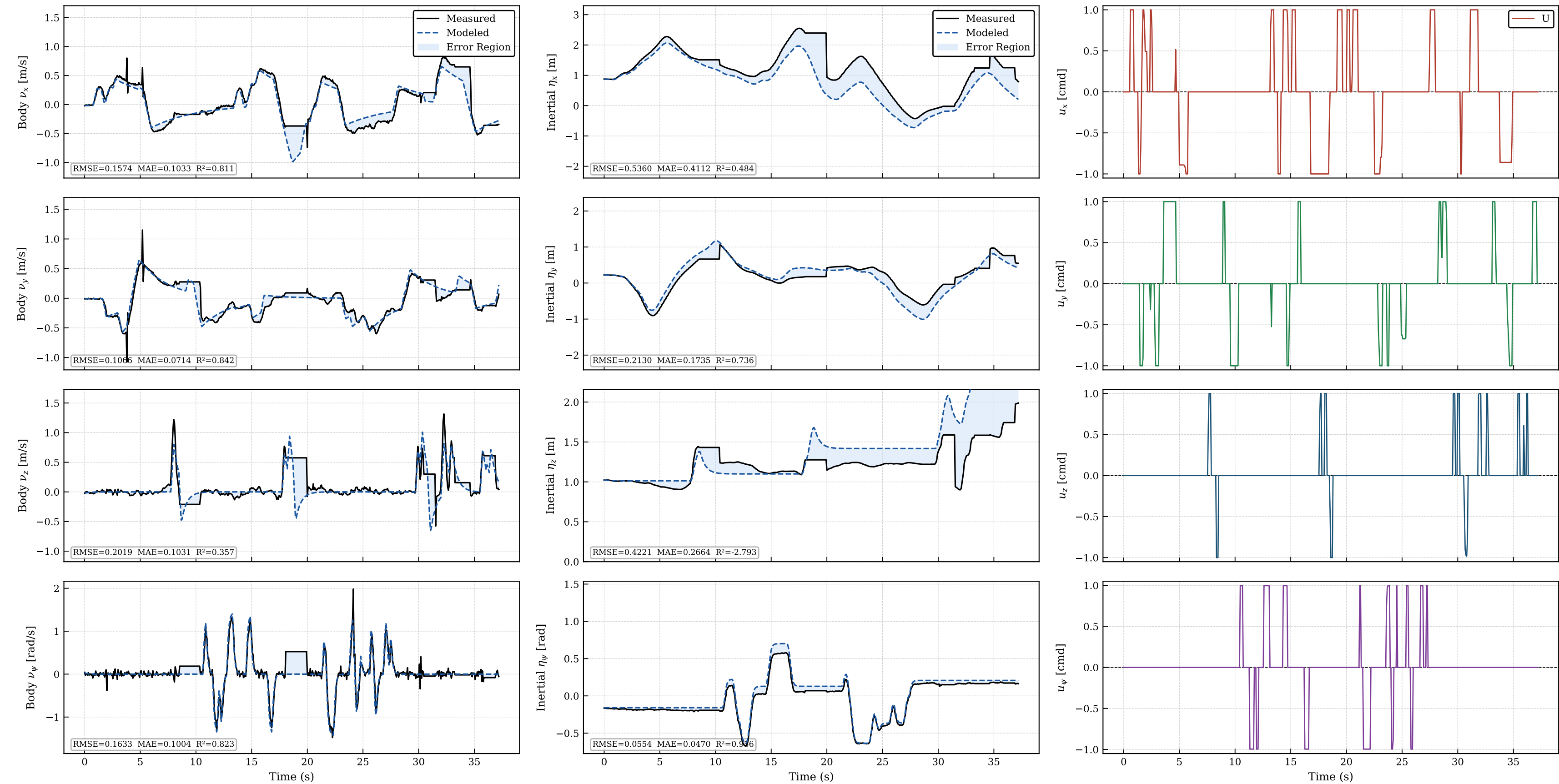
Validation — coupled_sine_joystick_09_Aug_2026_11h46min_B10_15Hz_COMPLETO.csv
