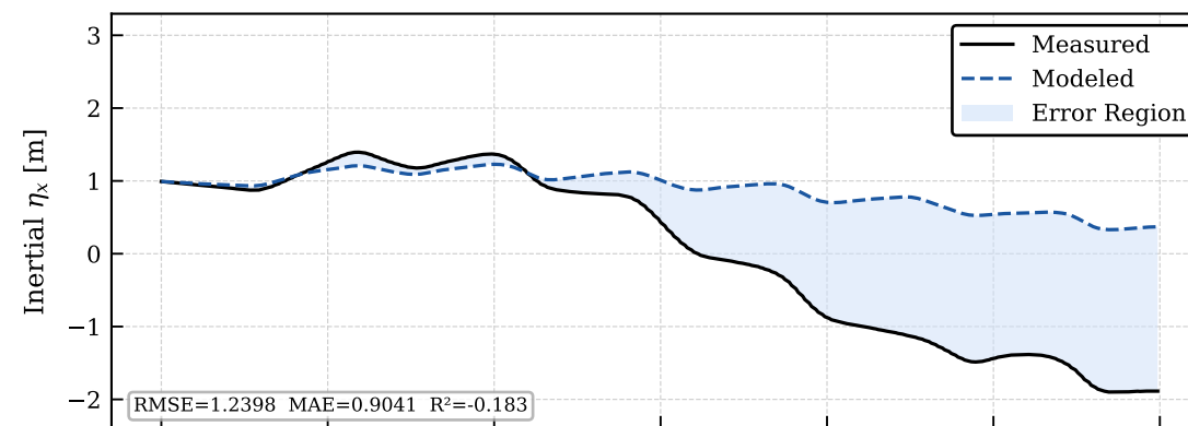
Validation — coupled_sine_ud_all_09_Aug_2026_11h36min_B10_15Hz_COMPLETEO.csv
