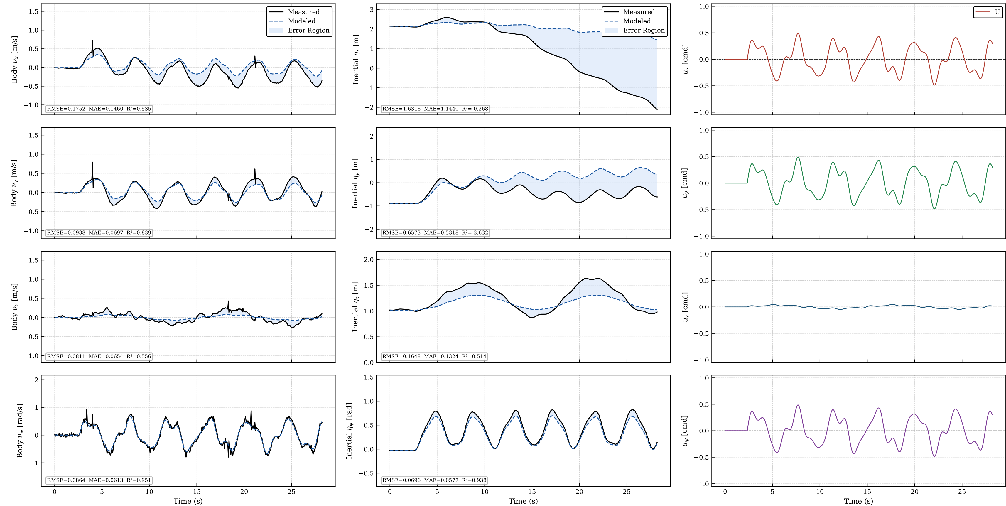
Validation — coupled_sine_ud_all_09_Aug_2026_11h41min_B10_15Hz_COMPLETEO.csv
