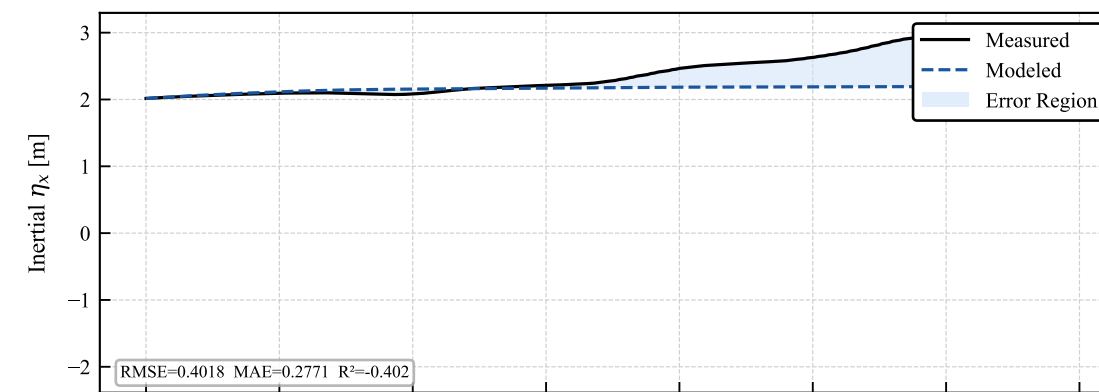
Validation — uncoupled_sine_udPsidot_09_Aug_2026_11h32min_B10_15Hz_COMPLETO.csv
