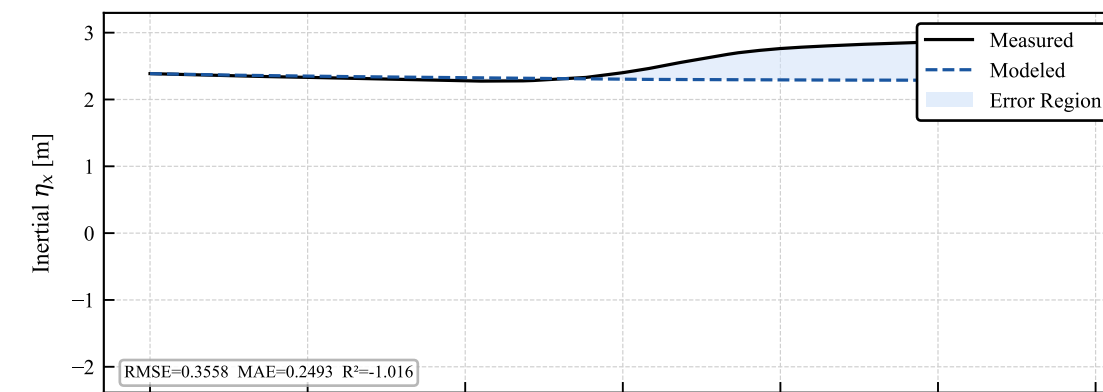
Validation — uncoupled_sine_udPsidot_08_Aug_2026_17h09min_B10_15Hz_COMPLETO.csv
