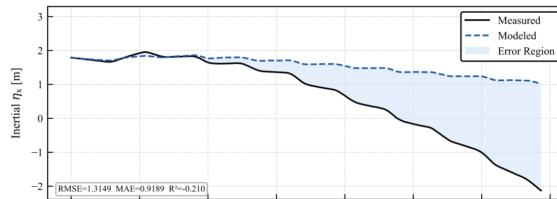
Validation — coupled_sine_ud_all_08_Aug_2026_17h14min_B10_15Hz_COMPLETO.csv
