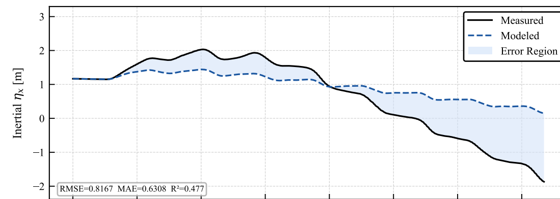
Validation — coupled_sine_ud_all_09_Aug_2026_11h40min_B10_15Hz_COMPLETO.csv
