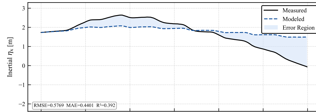
Validation — coupled_sine_ud_all_08_Aug_2026_17h15min_B10_15Hz_COMPLETO.csv
