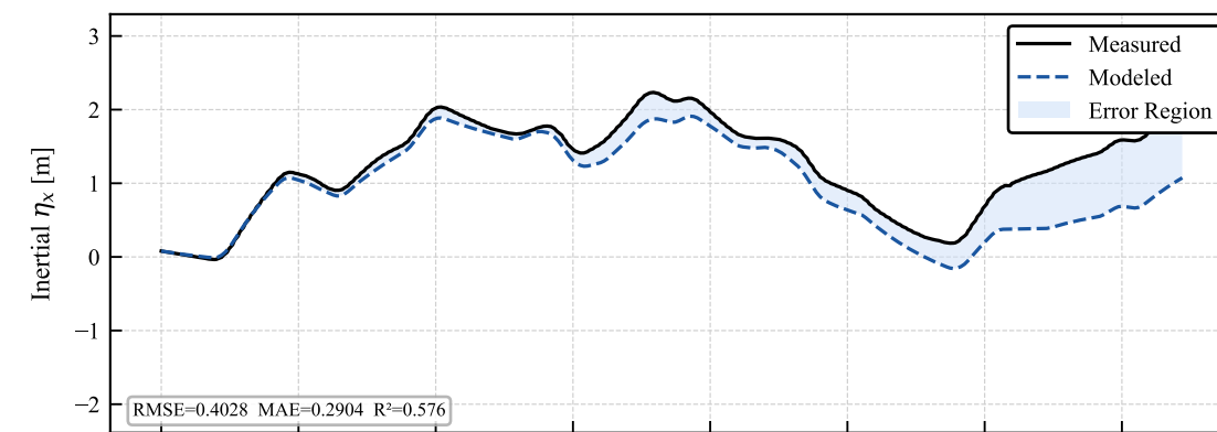
Validation — coupled_sine_joystick_09_Aug_2026_11h48min_B10_15Hz_COMPLETO.csv
