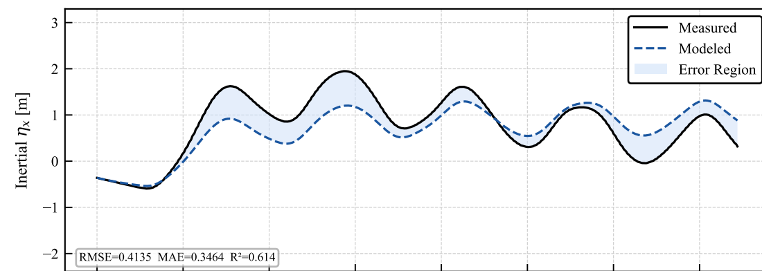
Validation — uncoupled_sine_udTheta_09_Aug_2026_11h14min_B10_15Hz_COMPLETO.csv
