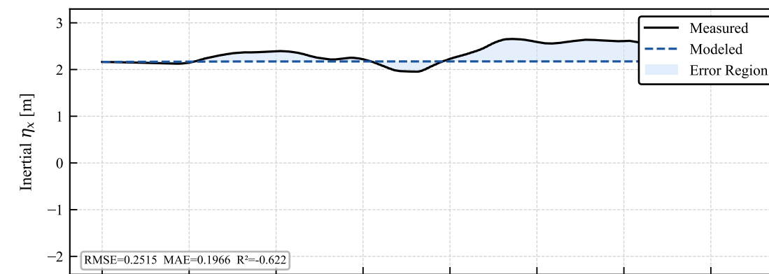
Validation — uncoupled_sine_udPsidot_09_Aug_2026_11h35min_B10_15Hz_COMPLETO.csv
