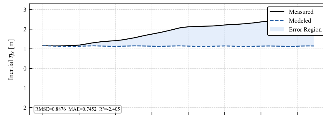
Validation — uncoupled_sine_udPhi_09_Aug_2026_11h22min_B10_15Hz_COMPLETO.csv
