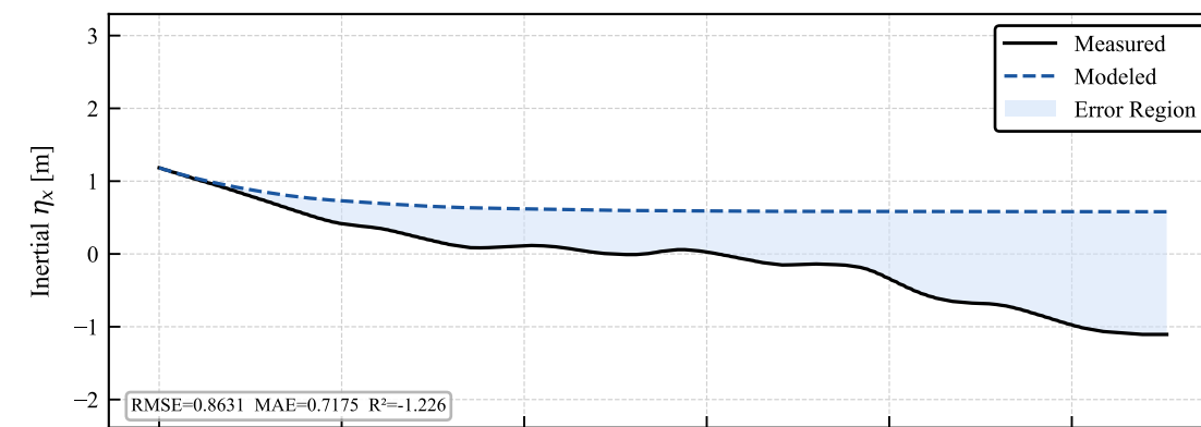
Validation — uncoupled_sine_udPsidot_09_Aug_2026_11h33min_B10_15Hz_COMPLETO.csv
