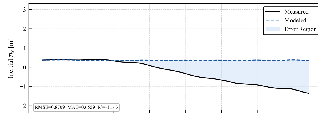
Validation — uncoupled_sine_udPhi_09_Aug_2026_11h18min_B10_15Hz_COMPLETO.csv
