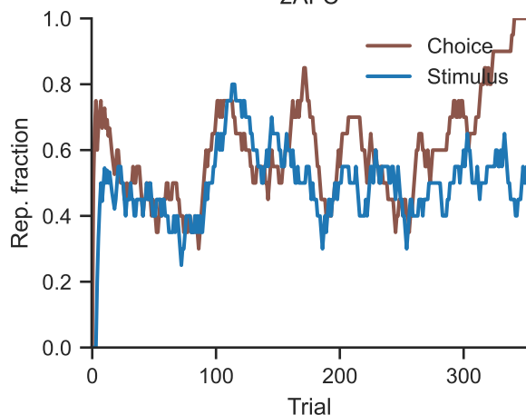
2AFC
