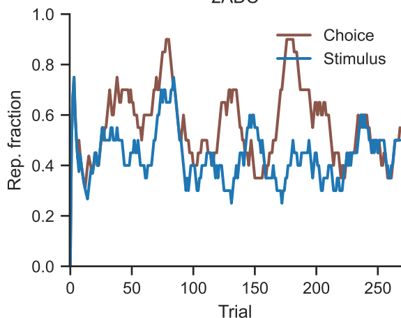
2ADC
