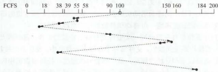
图 4-25 FCFS 磁盘调度算法
