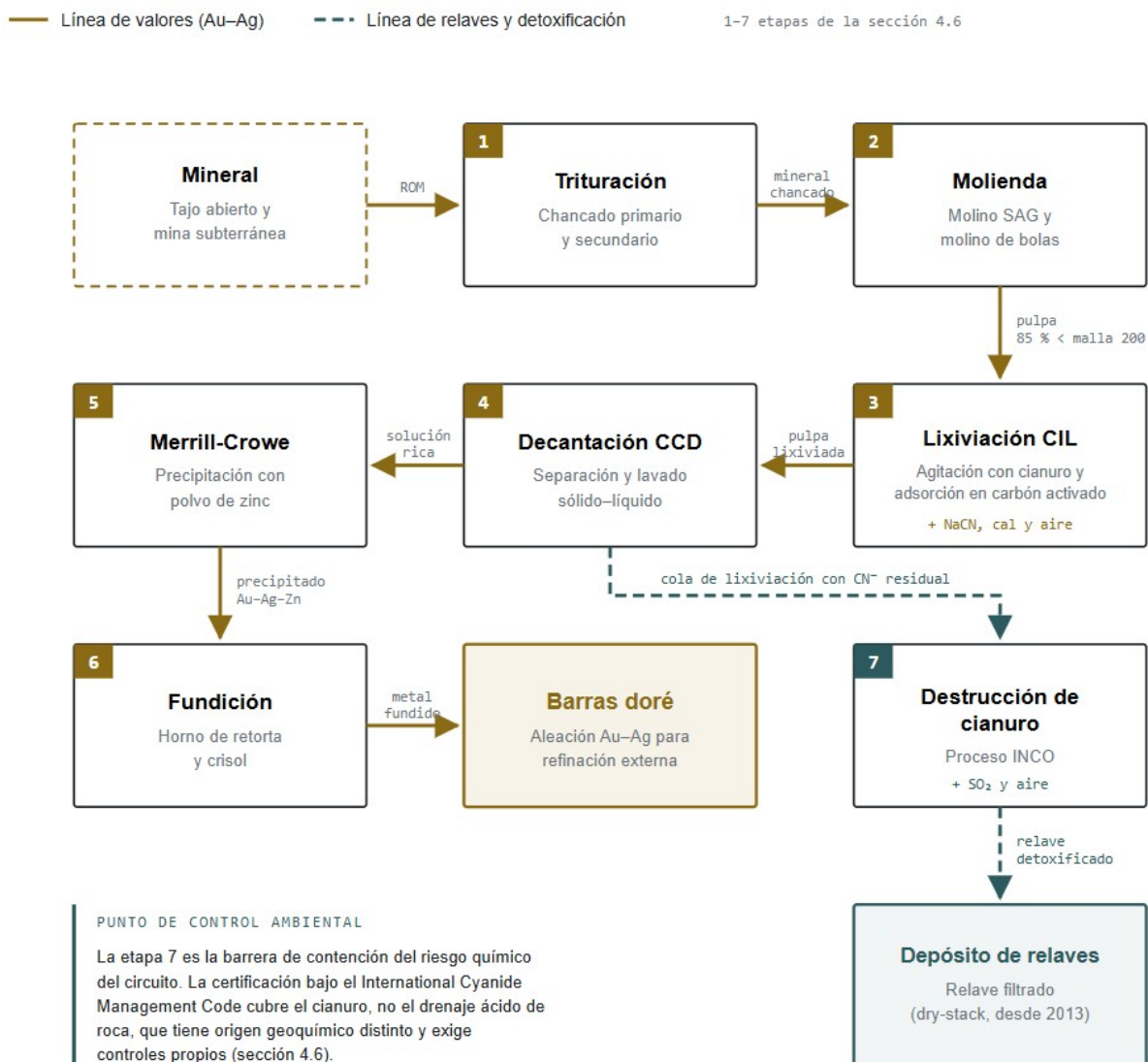
Figura 4.2: Diagrama de flujo del proceso metalúrgico de la Mina Marlin
