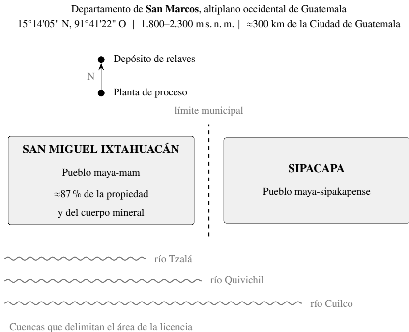
Figura 4.1: Esquema de ubicación de la Mina Marlin y de su entorno hidrográfico
