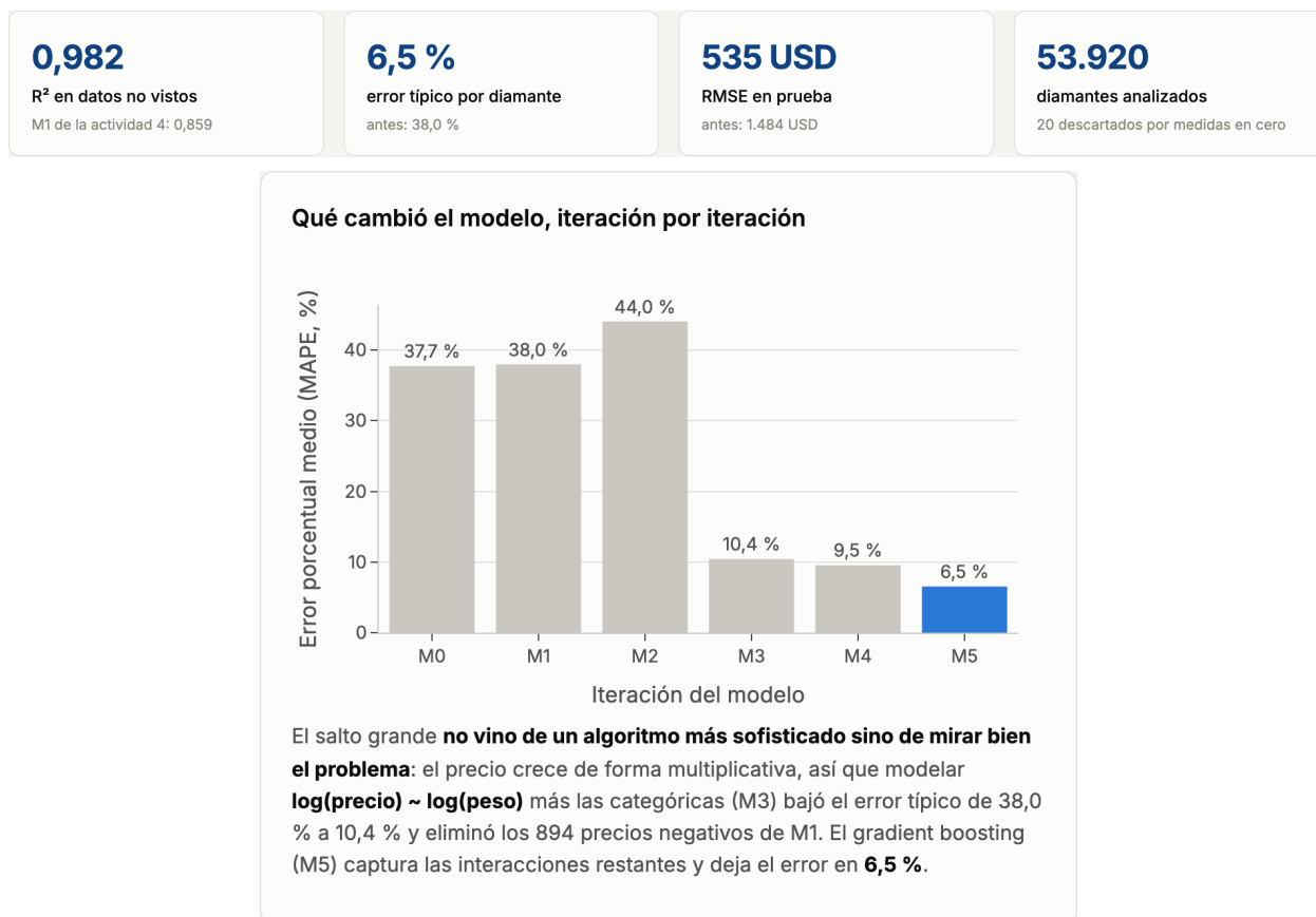
Figura 4. Pestaña 1: indicadores y evolución del error en cada iteración.
