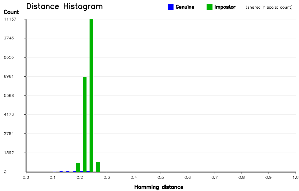
Rysunek 4: Histogram odległości Hamminga dla par genuine i impostor na MMU.
