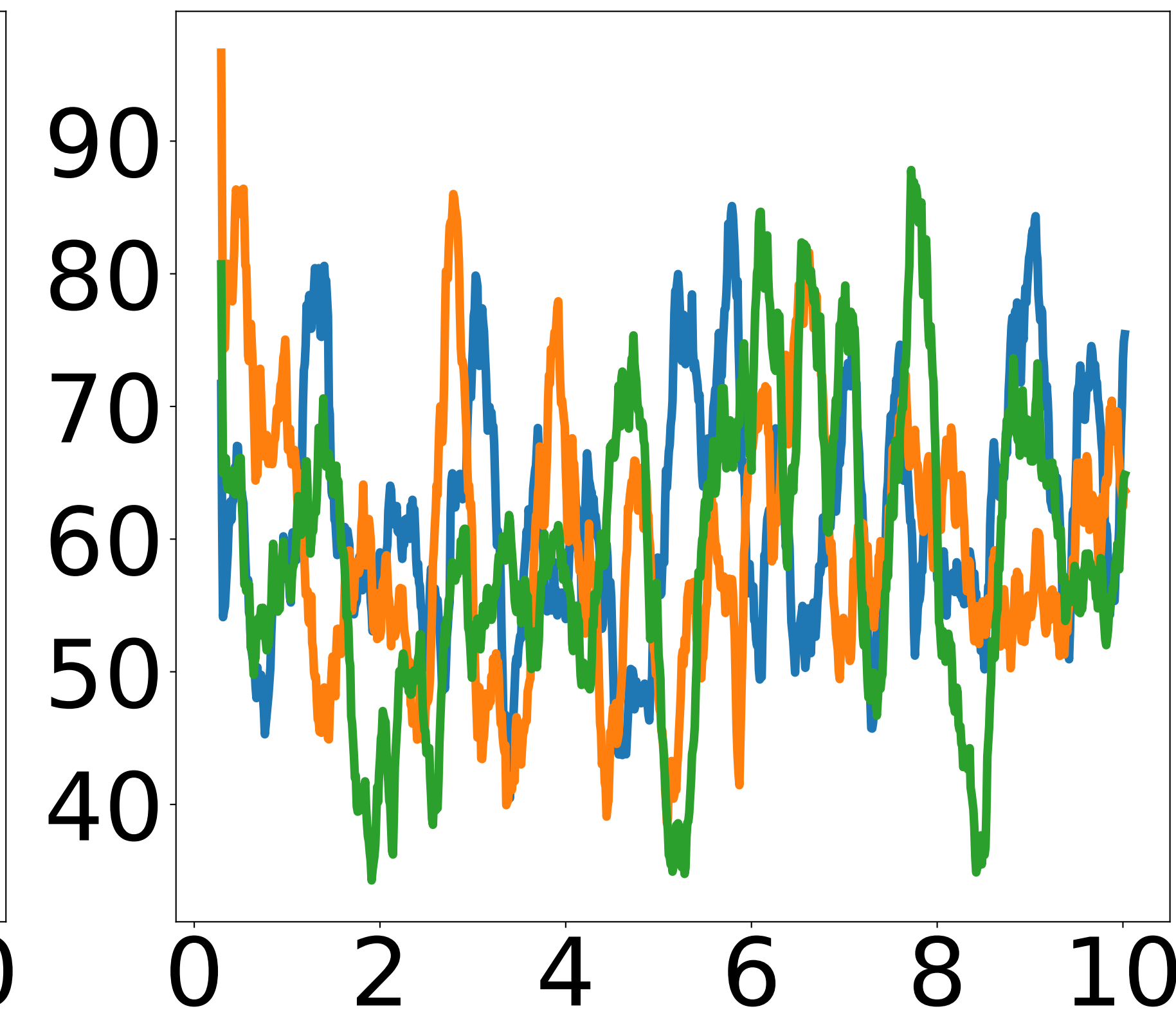
Tetracosanethiol
