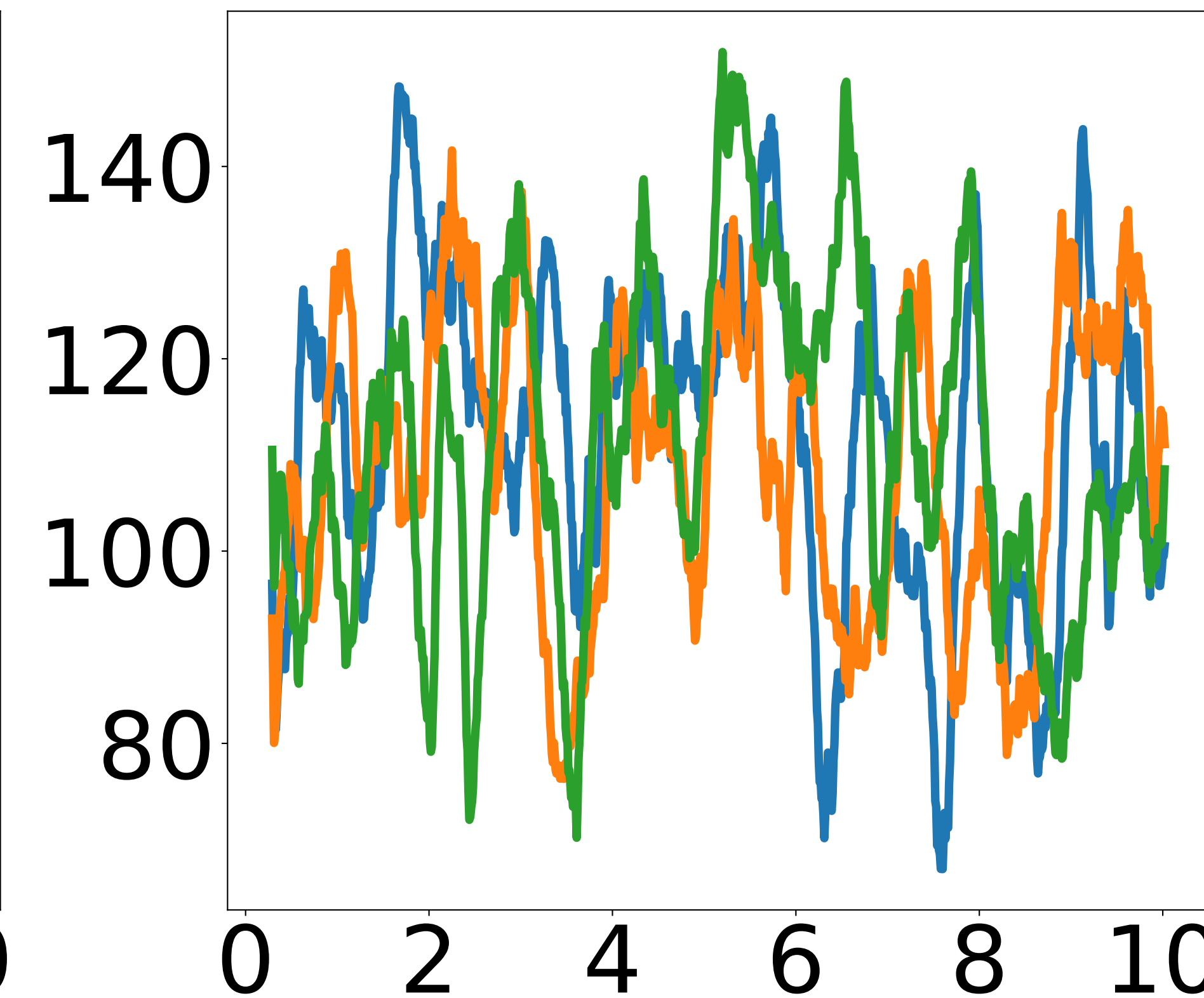
Icosanethiol
