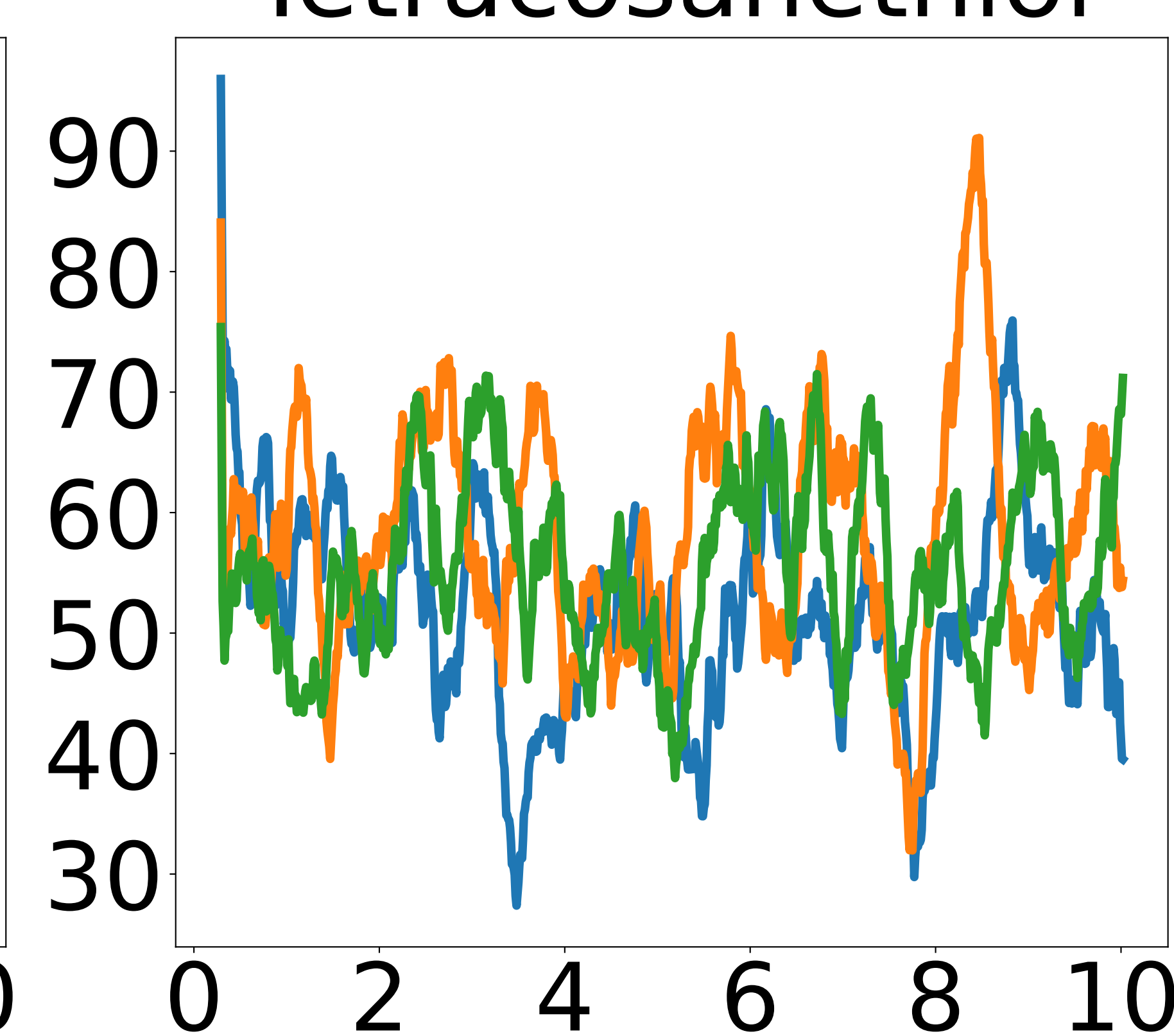
Tetracosanethiol
