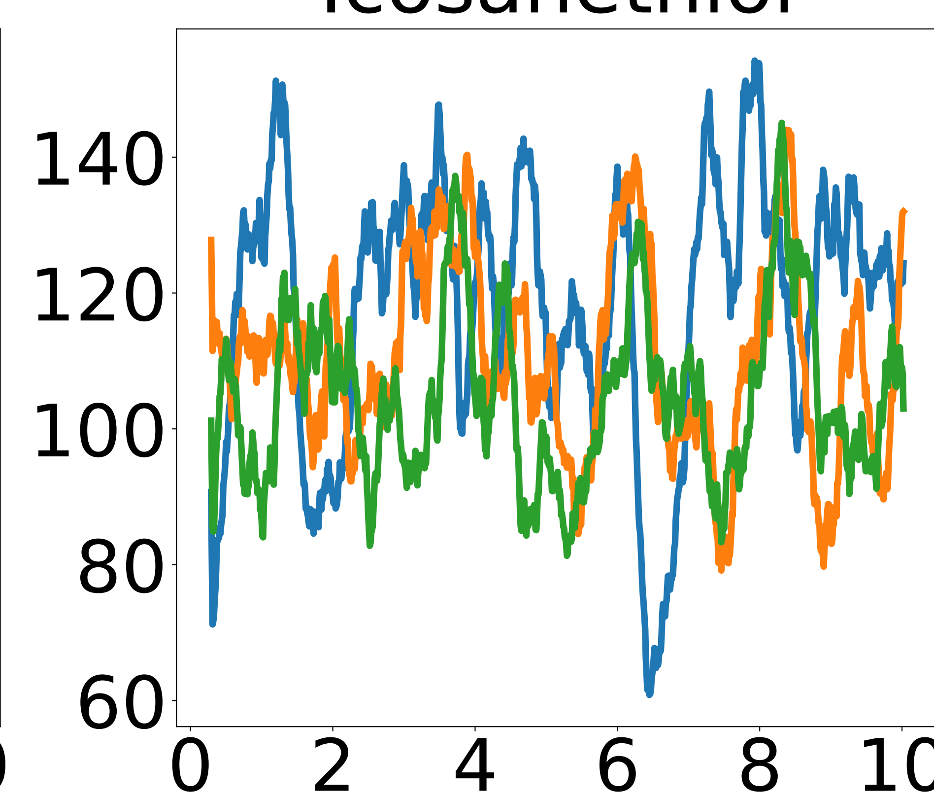
Icosanethiol
