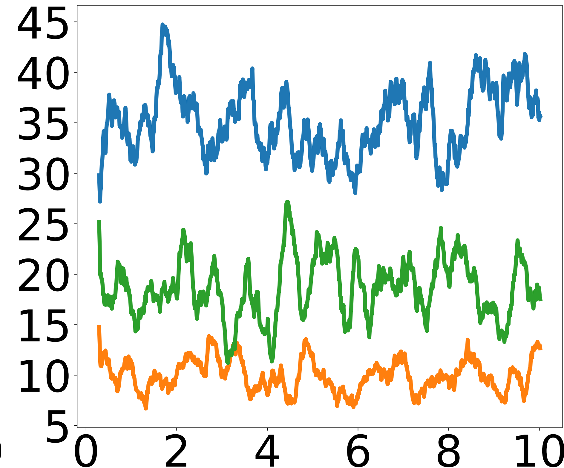
Icosanethiol
