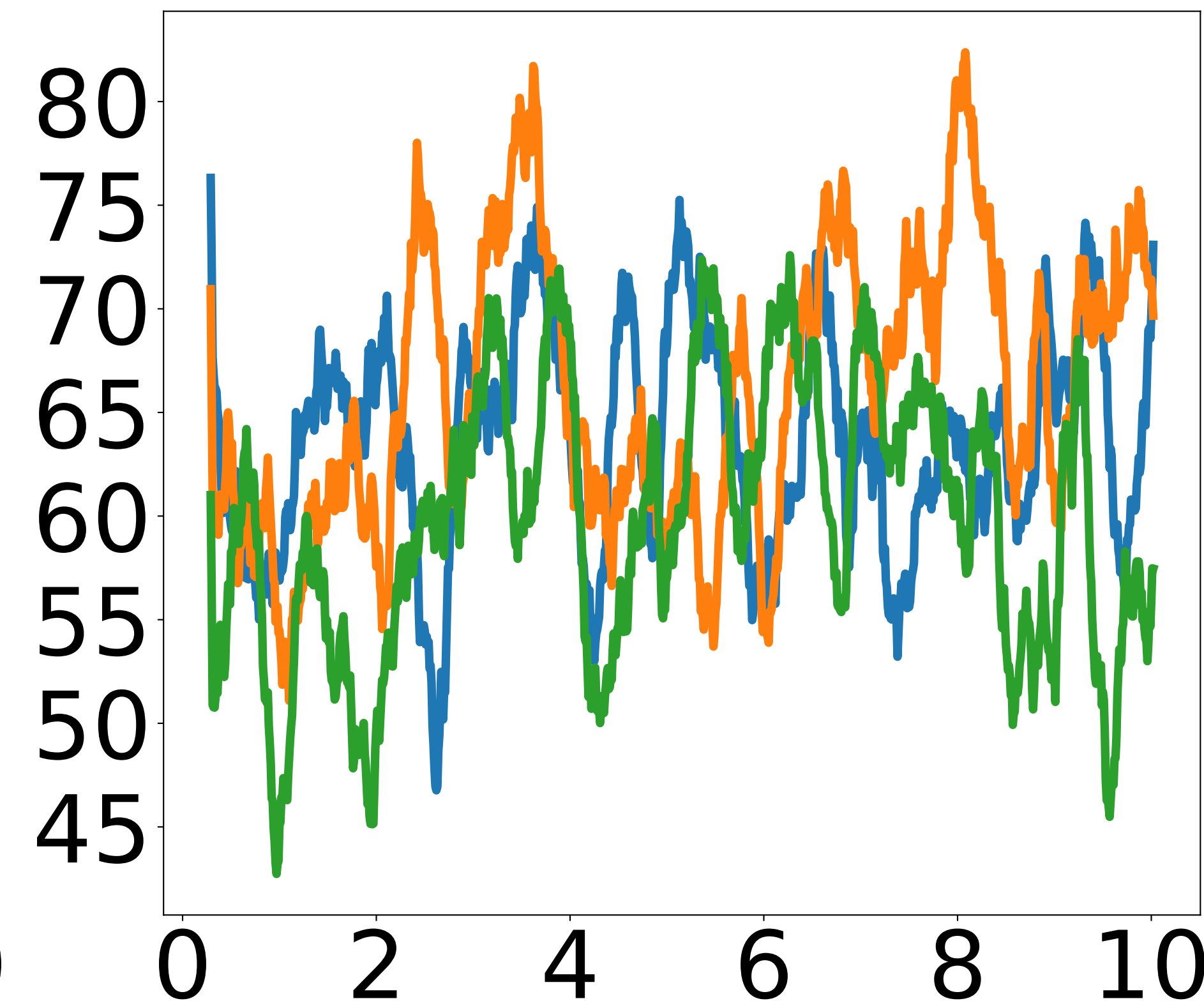
Tetracosanethiol
