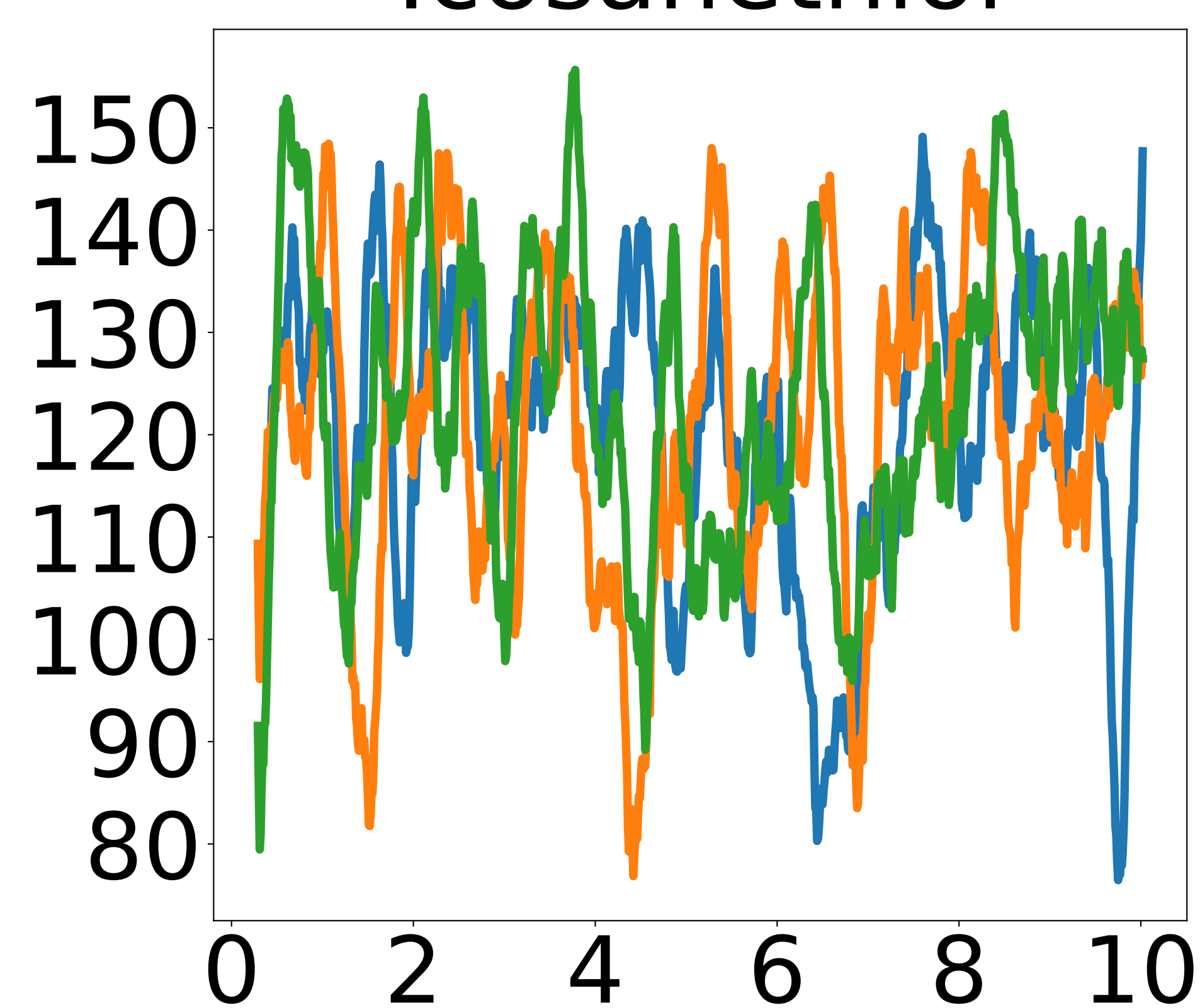
Icosanethiol
