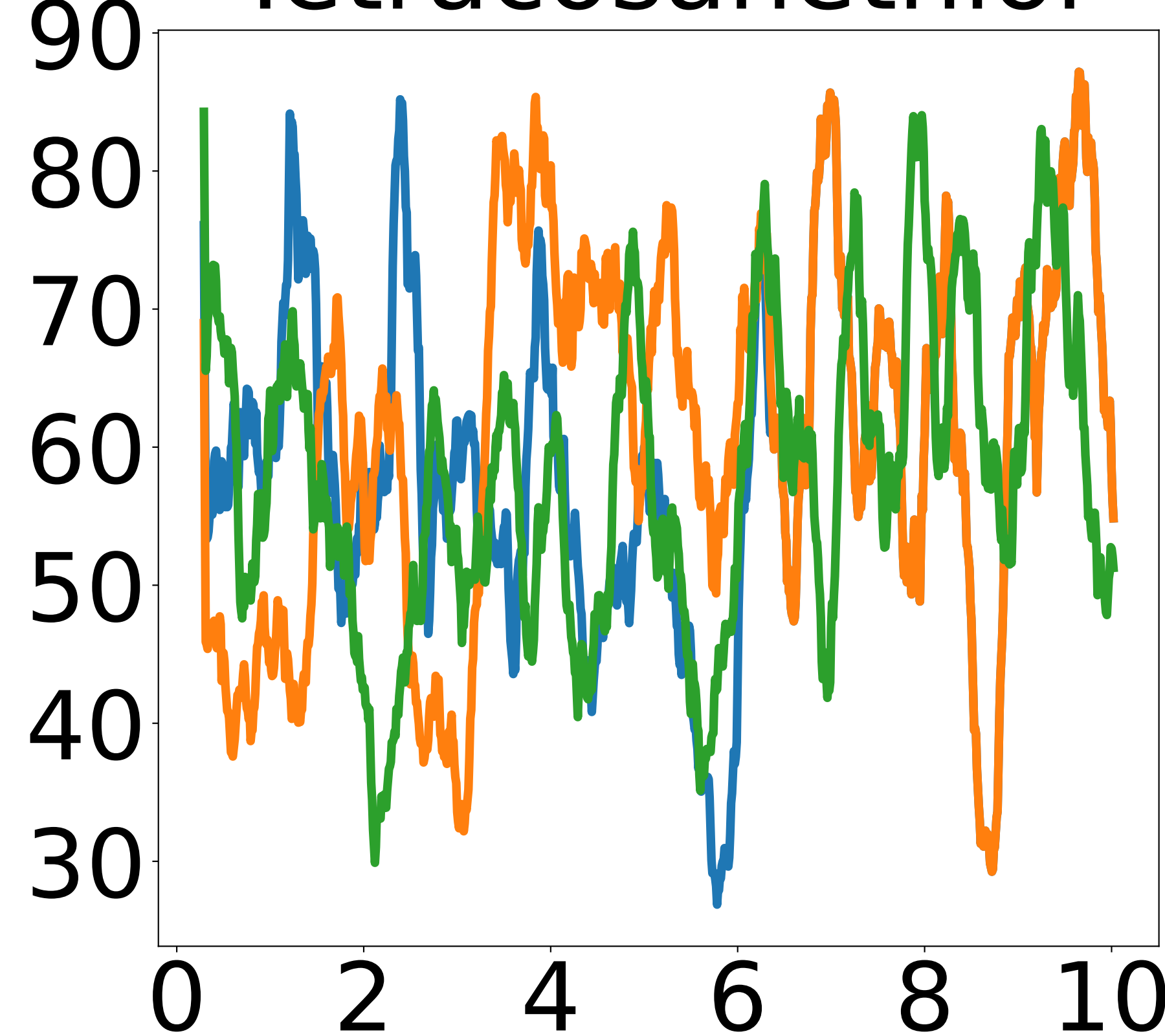
Tetracosanethiol
