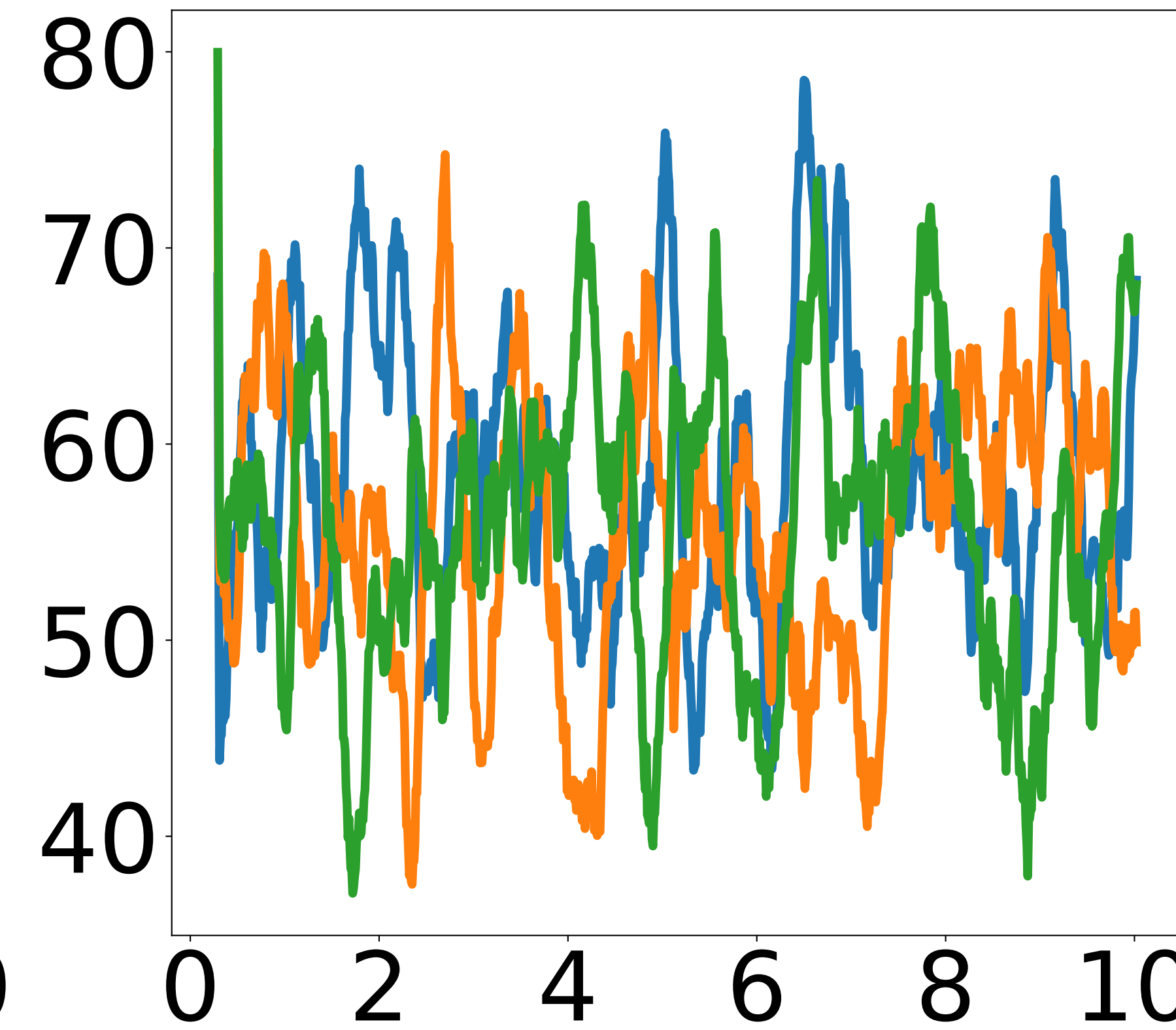
Tetracosanethiol
