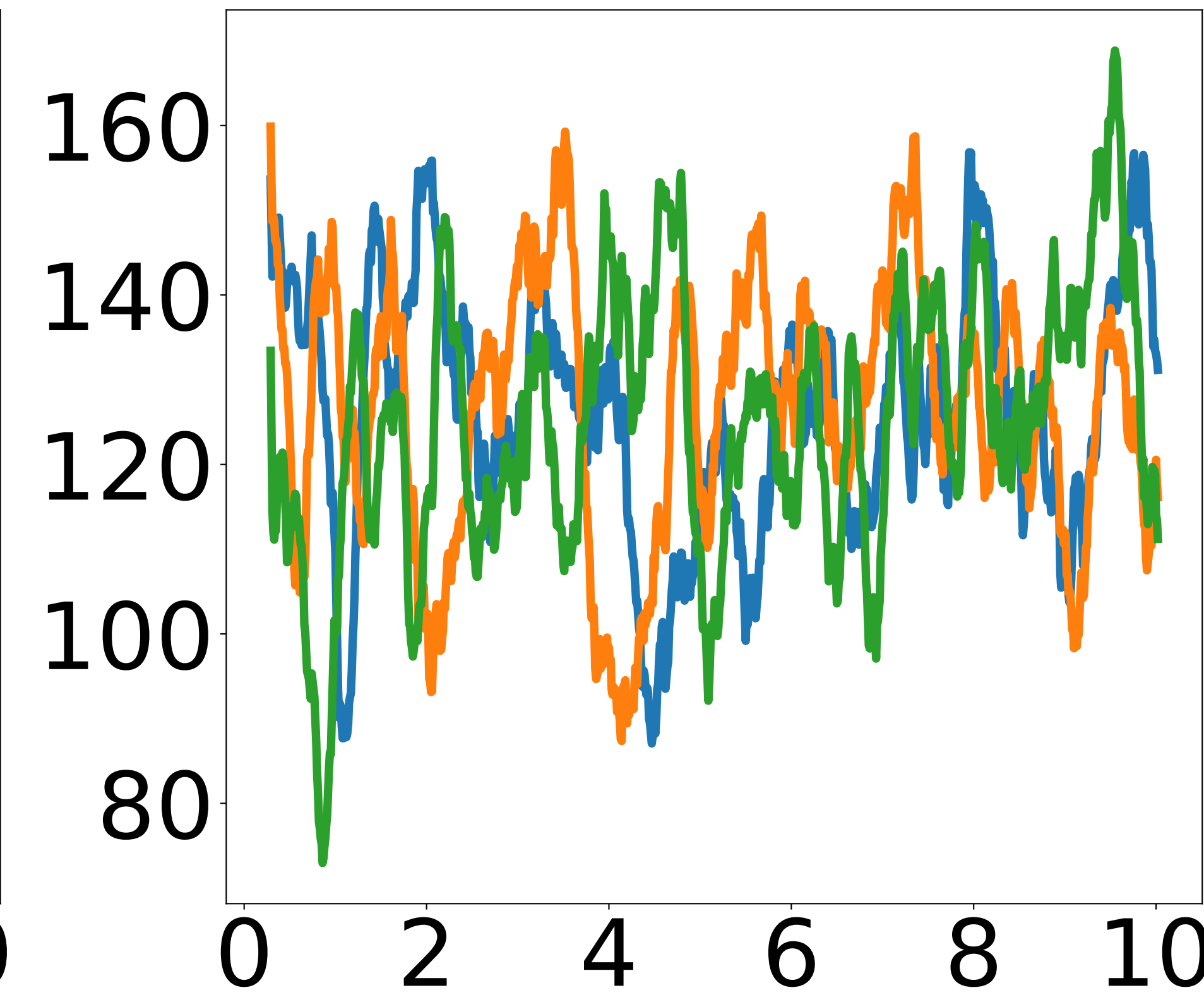
Icosanethiol
