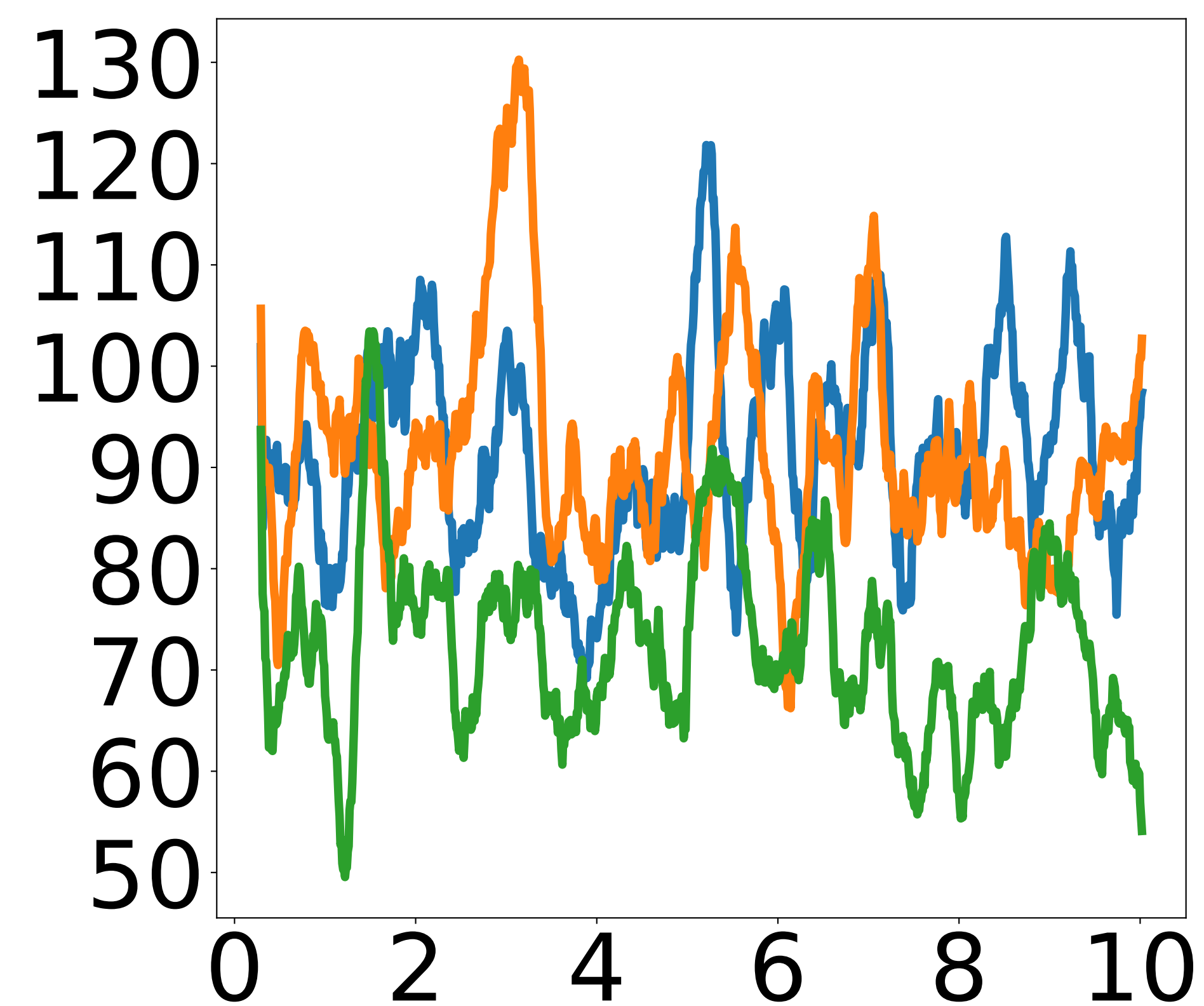
Icosanethiol
