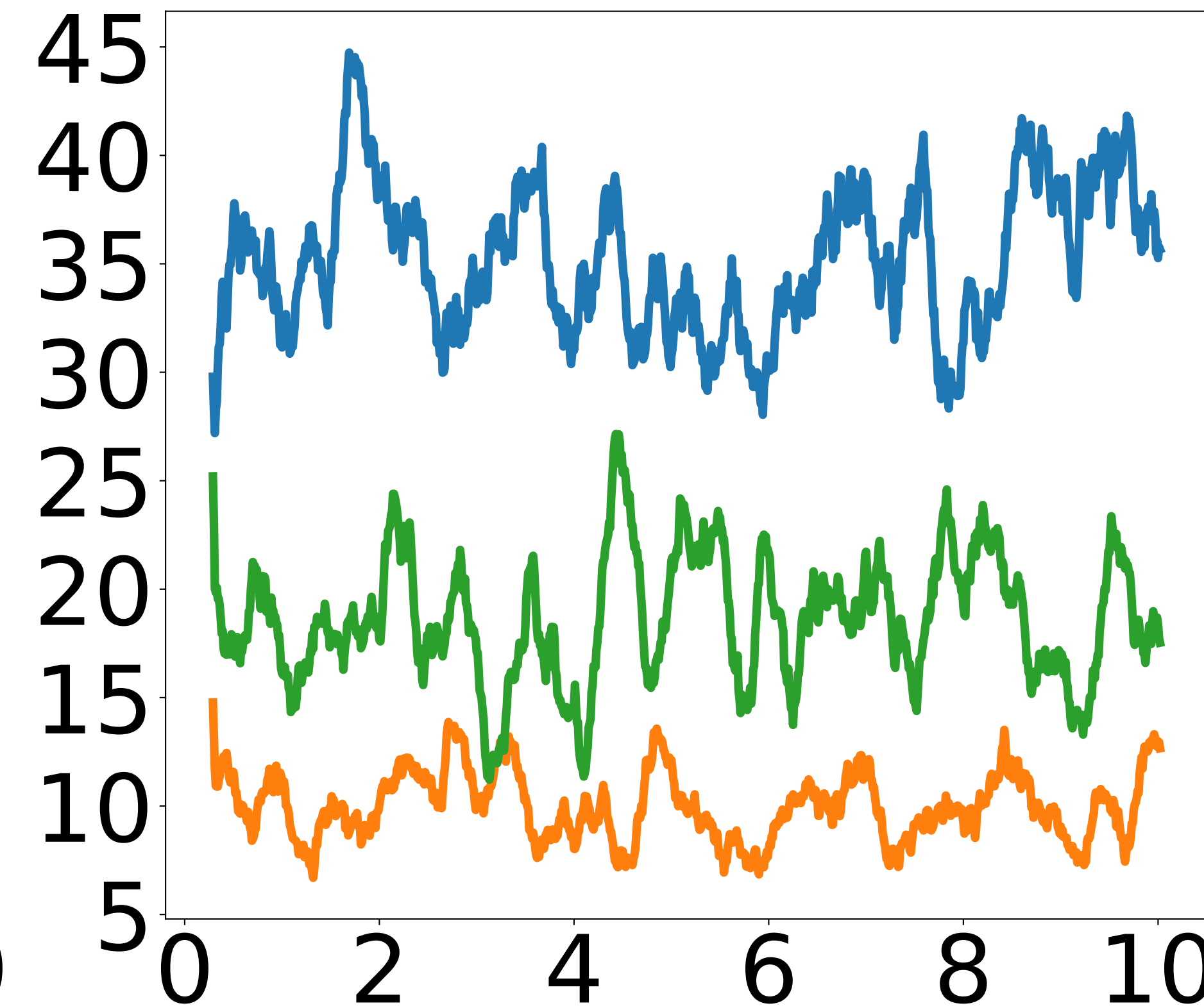
Icosanethiol
