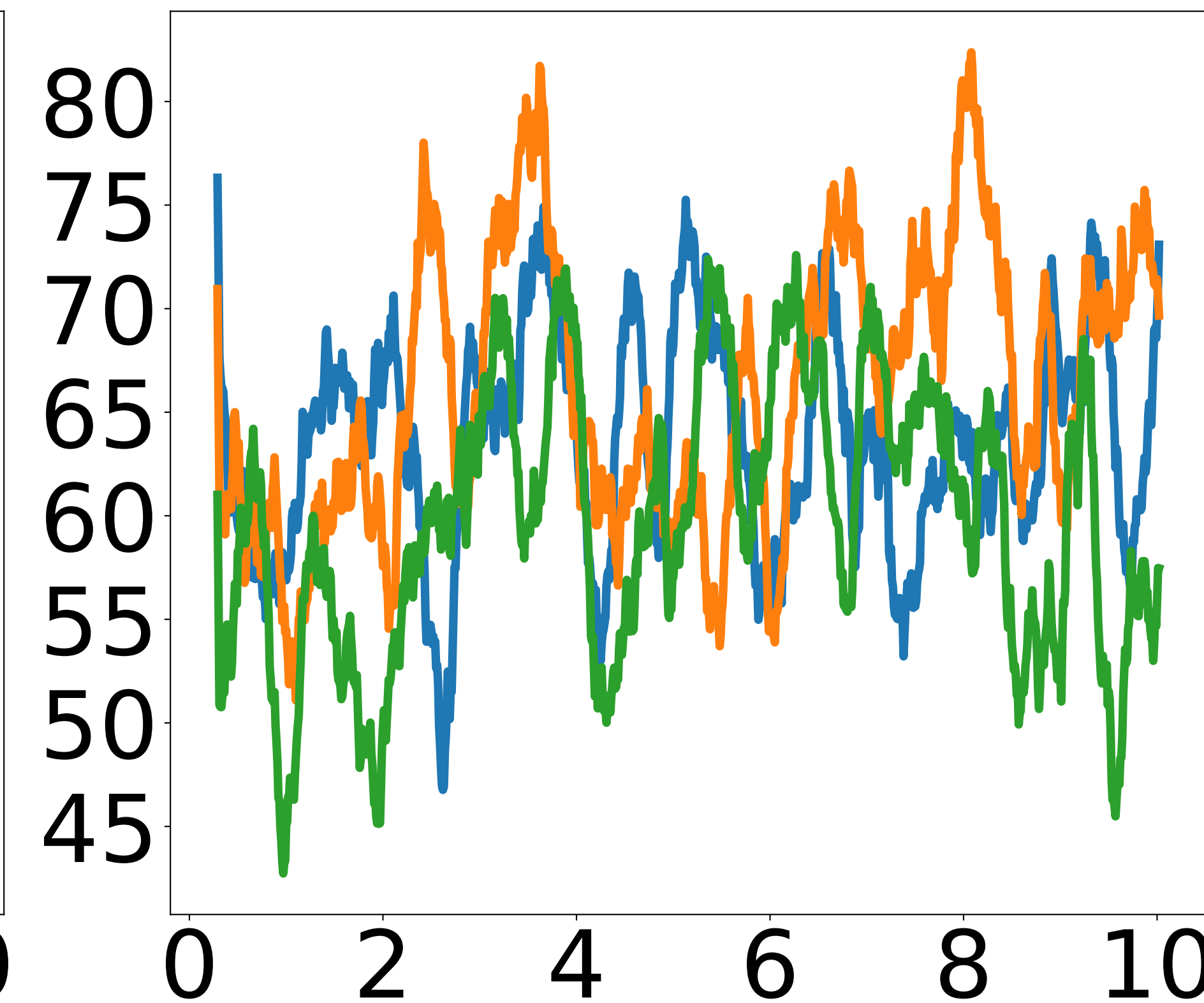
Tetracosanethiol
