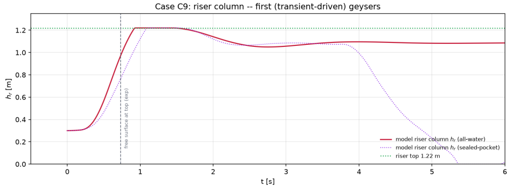
图 14: C9 竖管水柱高度 h_r : 全水变体 (实线) 与密闭气囊变体 (点线)。竖虚线标记试验第一阶段中水面首次到达竖管顶的时刻。
