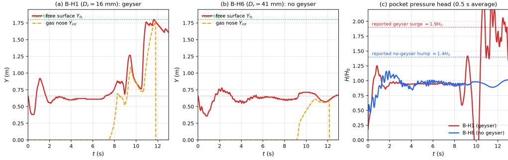
图 8: 算例组 2, [3] 签名工况 (全同步耦合): (a) 喷发工况 B-H1 ( D_r = 16 mm) 计算的竖管自由水面与气核前端轨迹; (b) 不喷发工况 B-H6 ( D_r = 41 mm) 同图; (c) 两工况计算的气囊压头 (0.5 s 平均) 与文献报告峰值水平对比 (喷发涌峰 \approx 1.9 H_0 ; 不喷发隆起 \approx 1.4 H_0 )。
