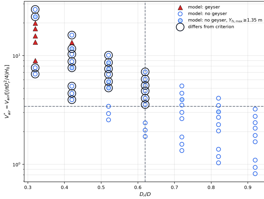
图 9: 算例组 2: 覆盖 [3] 试验参数范围 ( D_r = 16\text{--}46\text{ mm} , L_0 = 0.61\text{--}1.8\text{ m} , H_0 = 0.66\text{--}0.88\text{ m} ) 的 63 个构型的模型喷发分类, 每个均为一次全同步模拟, 绘于式 (11) 的判据平面。实心三角: 模型喷发; 空心圆: 模型不喷发 (浅色实心圆: 水面到管顶 0.45 m 以内); 黑圈: 与判据分歧; 虚线: 判据阈值 D_r/D = 0.62 与 V_{air}^* = 3.42 。模型在 63 个构型中的 39 个上一致; 全部 24 处分歧均为判据判喷/模型判不喷, 无一例假阳性。
