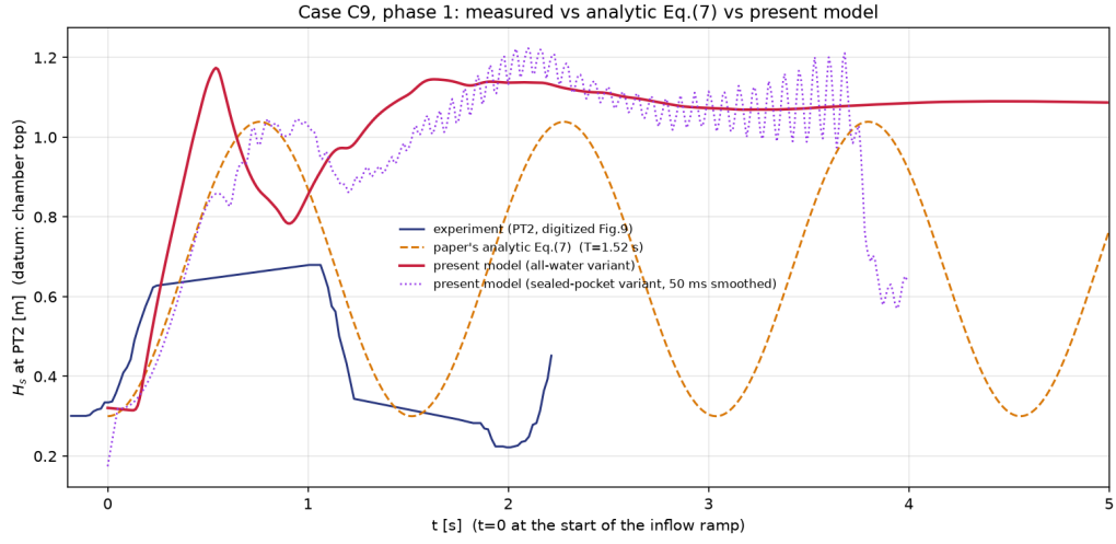
图 13: C9 第一阶段 ( t < 5 s): 交汇室顶盖基准下的 PT2 水头 H_s 。蓝色: 从 [5] 图 9 数字化的试验值; 橙色虚线: 文献式 (7); 红色: 本文全水模型; 紫色点线: 密闭气囊变体 (50 ms 平滑)。气囊于 t \approx 6.5 s 抵达后的气囊驱动喷发未计算。
