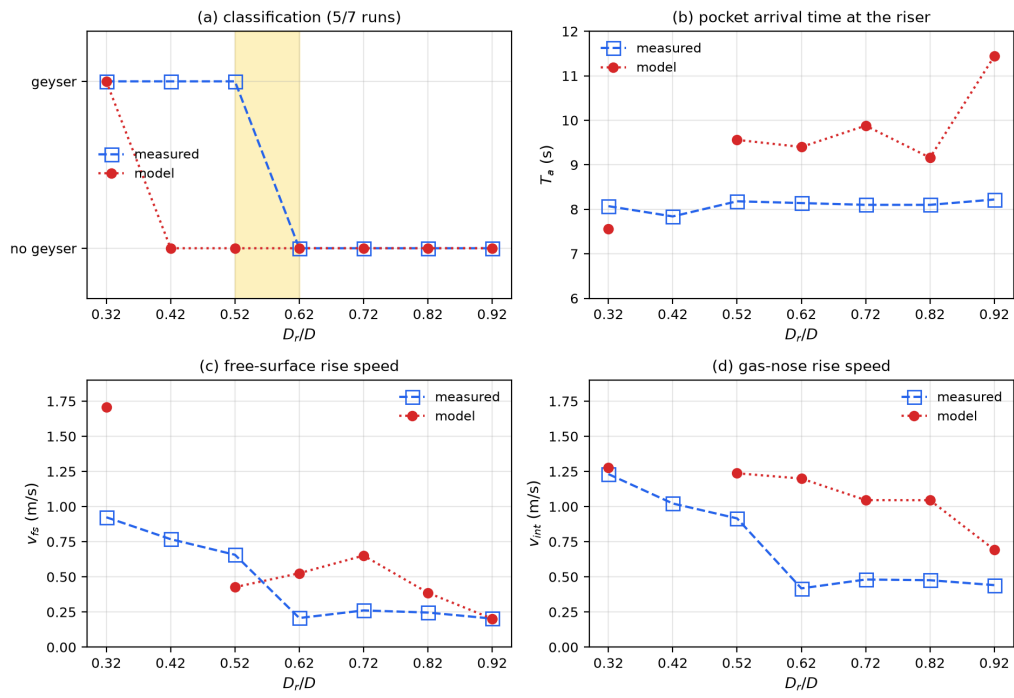
图 7: 算例组 2, [3] Series B: 实测与计算的 (a) 喷发分类, (b) 气囊到达竖管时间, (c) 水面平均上升速度, (d) 气核前端平均上升速度, 均以竖管-管道直径比 D_r/D 为横轴。
