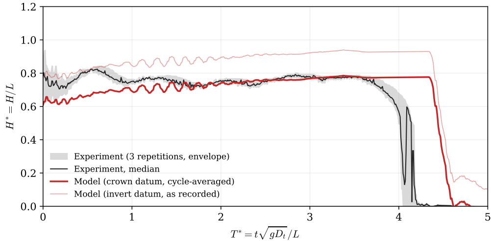
图 5: Test B ( D_t/D = 0.135 , H_{a0} = 0.610 m, Y_{fs,0} = 0.356 m): 传感器压头 H^* 随 T^* 变化。灰色带与深色线: [2] 图 6 三次试验重复的数字包络与中位线; 红色粗线: 模型压头 (0.4 s 窗口周期平均, 管顶基准, 即传感器测点与塔基高程, 相对管底记录 -D/L ); 红色浅线: 同一迹线的管底基准原始记录。
