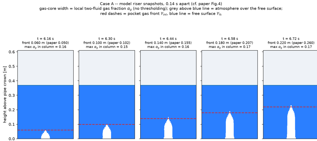
图 4: Test A: 气水界面爬升期间以 0.14\text{ s} 间隔输出的塔内计算快照 (对照 [2] 图 4 摄影序列)。蓝: 水; 白: 气核 (当地两流体气体分数); 灰: 自由水面上方大气。红色虚线为计算的气囊前沿 Y_{int} ; 各栏标题给出模型与摄影的前沿高程。
