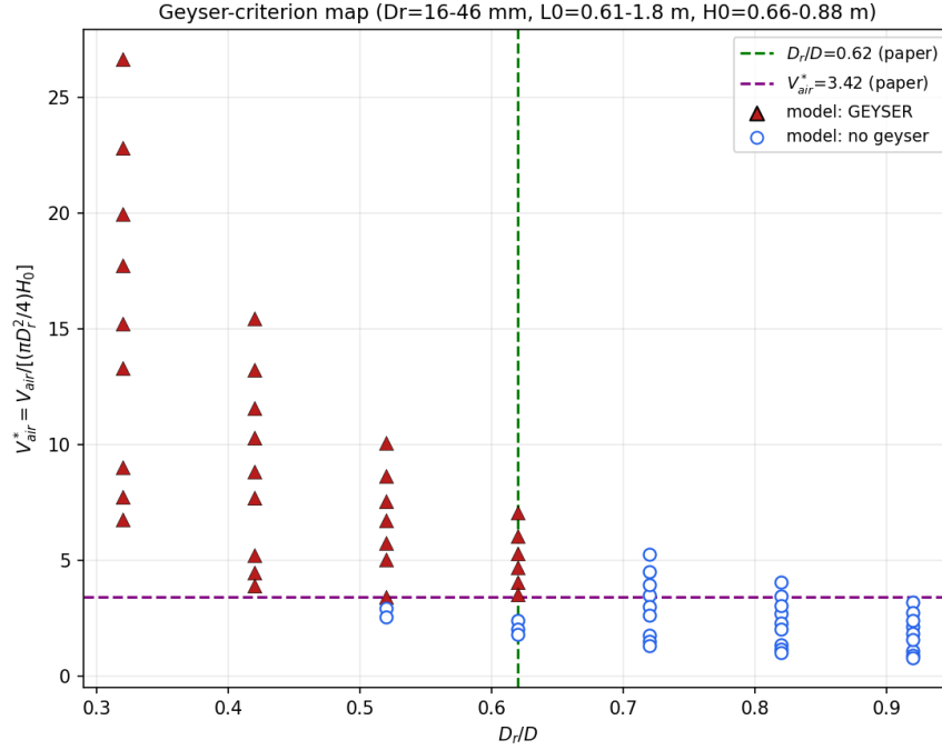
图 9: 算例组 2: 覆盖 [3] 试验参数范围 ( D_r = 16\text{--}46\text{ mm} , L_0 = 0.61\text{--}1.8\text{ m} , H_0 = 0.66\text{--}0.88\text{ m} ) 的 63 个构型的模型喷发分类, 绘于式 (7) 的判据平面。实心三角: 模型喷发; 空心圆: 模型不喷发; 虚线: 试验判据阈值 D_r/D = 0.62 与 V_{air}^* = 3.42 。模型与判据在 63 个构型中的 62 个上一致; 唯一分歧位于 V_{air}^* 阈值上 (3.418 对 3.42)。
