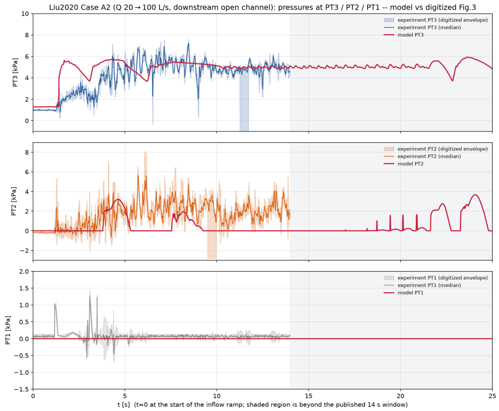
图 10: 工况 A2: 压力时程 (蓝: 数字化 Fig.3; 红: 模型)。
