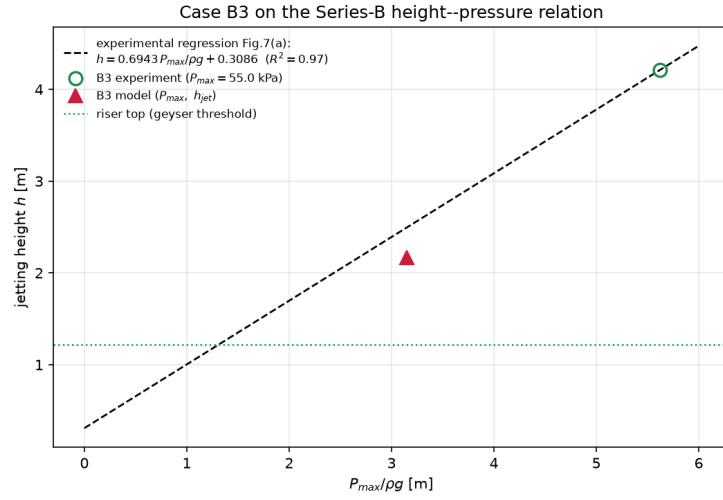
图 12: 工况 B3 在 Fig.7(a) h-P_{\max} 图上的落点 (红实心: 模型)。
