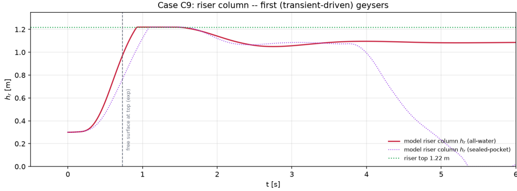
图 14: C9: 竖管水柱高度（全水实线、封气点线）。
