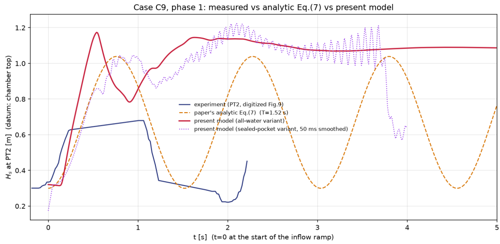
图 13: C9 第一阶段 ( t < 5 s): PT2 水头—试验、Eq.(7) 与全水模型。
