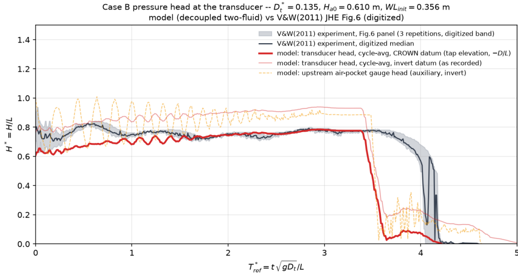
图 5: Test B ( D_t/D = 0.135 , H_{a0} = 0.610 m, Y_{fs,0} = 0.356 m): 传感器压头 H^* 随 T^* 变化。灰色带: [2] 图 6 数字化的 3 次试验重复; 深色线: 数字化中位线; 红色粗线: 模型压头 (0.4 s 窗口周期平均, 管顶基准, 即传感器测点与塔基高程, 相对管底记录 -D/L ); 红色浅线: 同一迹线的管底基准原始记录; 橙色虚线: 模型上游气囊表压头 (辅助量, 管底基准)。
