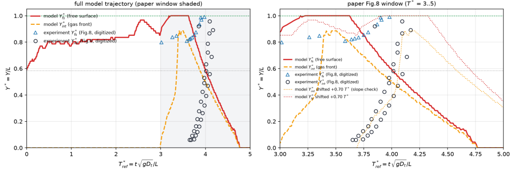
图 6: Test B: 塔内自由水面高程 Y_{fs}^* (红) 与气水界面高程 Y_{int}^* (橙, 虚线) 随 T^* 变化。左: 全程模型轨迹 (阴影为发表观测窗口)。右: 发表窗口 ( T^* = 3\text{--}5 ), 叠加 [2] 图 8 数字化试验散点 (三角: 水面; 圆圈: 界面); 点线为刚体平移 +0.70 个时间单位的模型轨迹, 用以把爬升运动学与管顶气穴系统性提前抵塔的影响分离。
