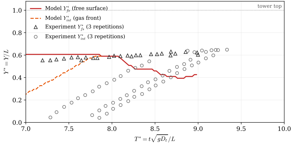
图 3: Test A: 文献发表观测窗口 ( T^* = 7-10 ) 内塔内自由水面高程 Y_{fs}^* (实线) 与气水界面高程 Y_{int}^* (虚线) 随 T^* 变化。散点为 [2] 图 7 数字化的三次试验重复 (三角: 水面; 圆圈: 界面)。模型气相前沿曲线画至其追上自由水面的时刻为止 (此后两界面合并, 不再存在独立前沿); 模型水面曲线画至实验数据覆盖范围为止。
