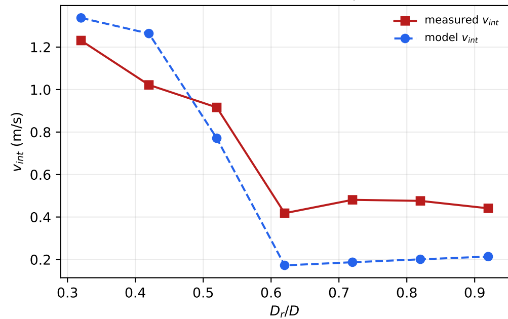
(d) Gas-nose mean rise speed
