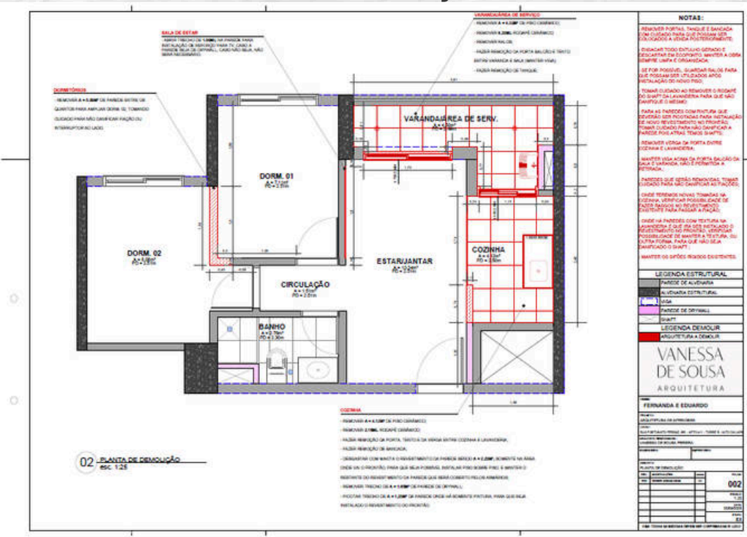
PLANTA DE DEMOLIÇÃO
