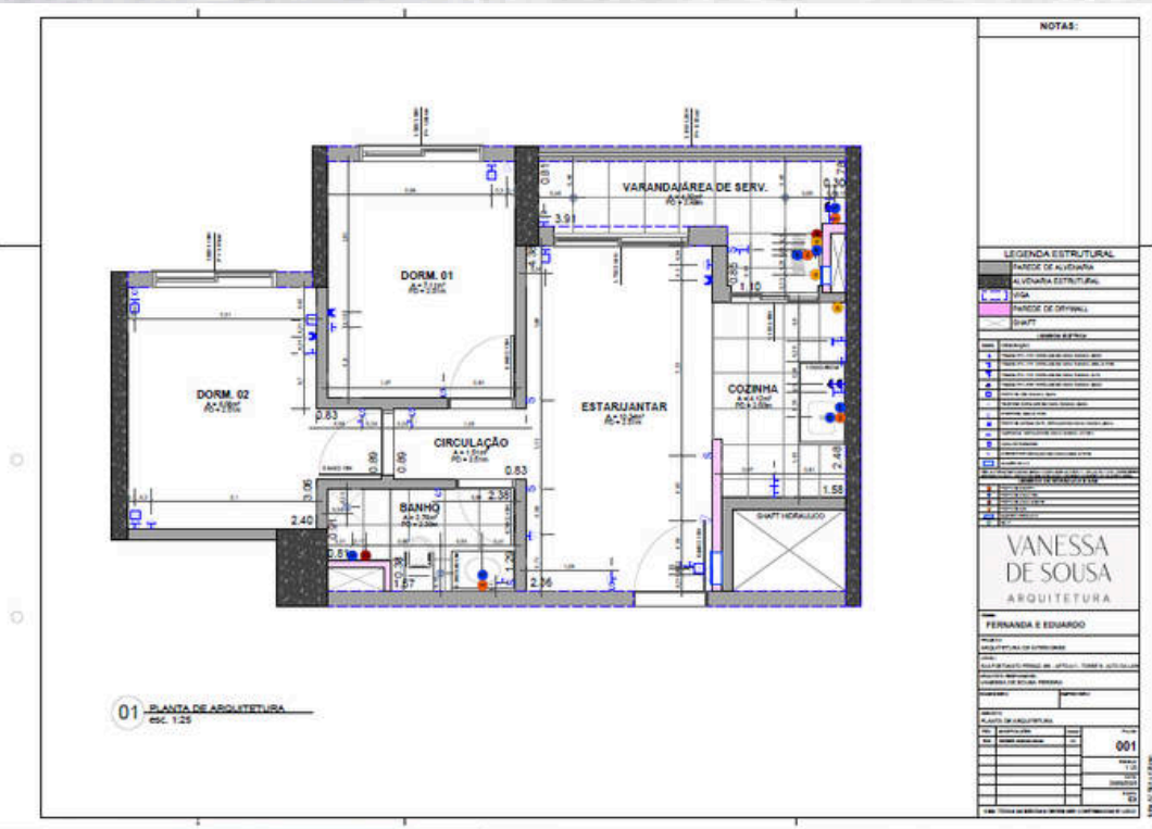
PLANTA DE ARQ.
