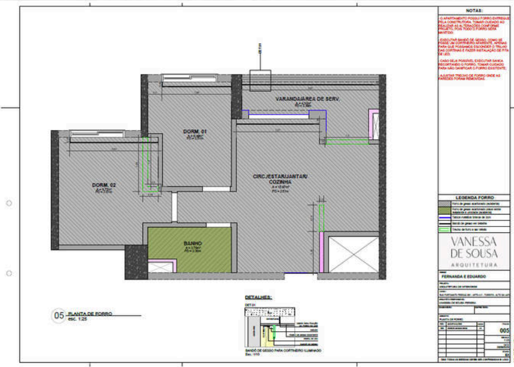
PLANTA DE FORRO
