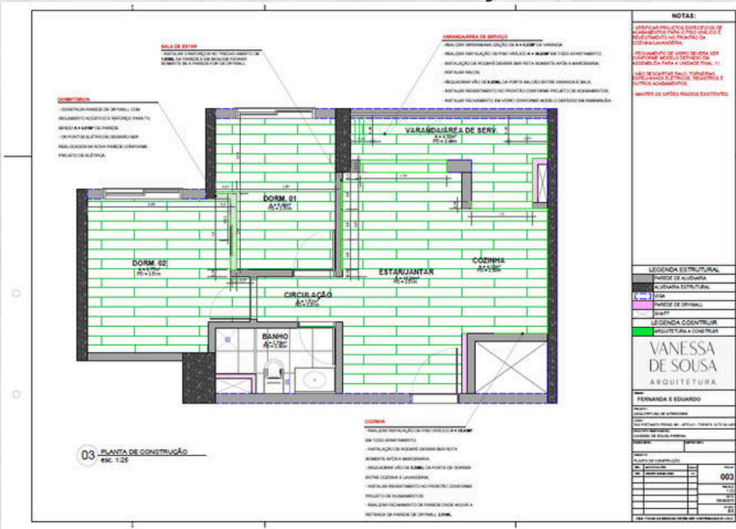
PLANTA DE CONSTRUÇÃO
