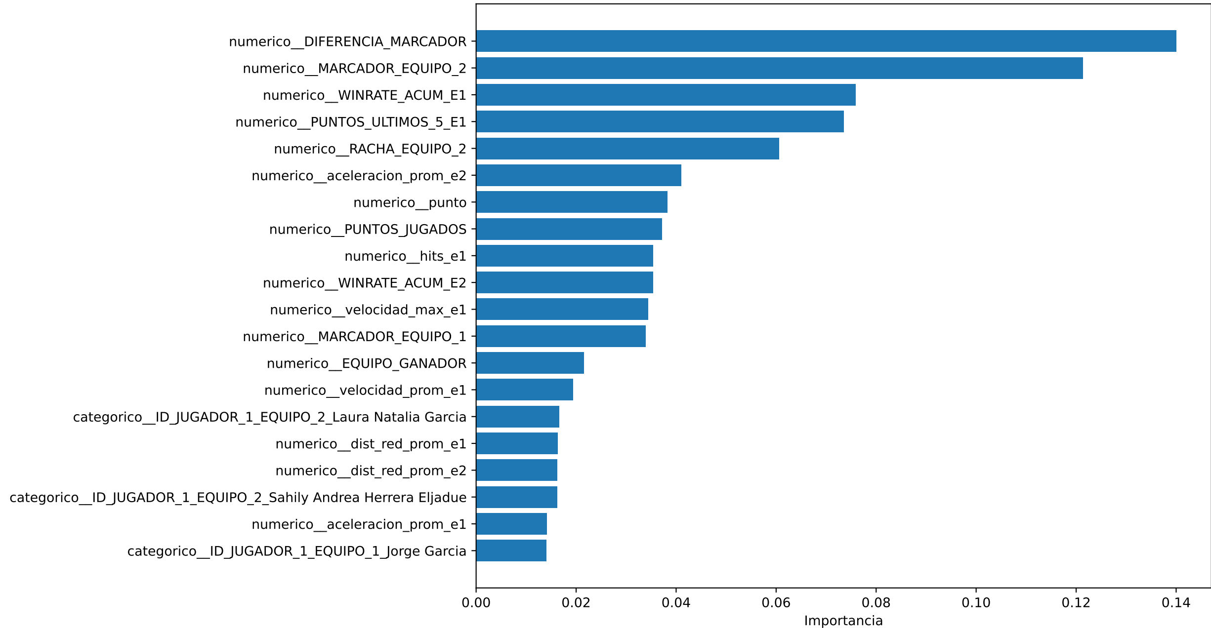
Top 20 Variables Más Importantes
