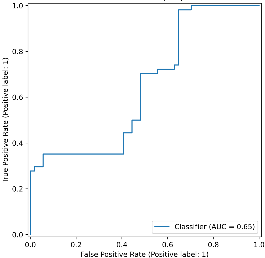
Curva ROC - holdout por partidos
