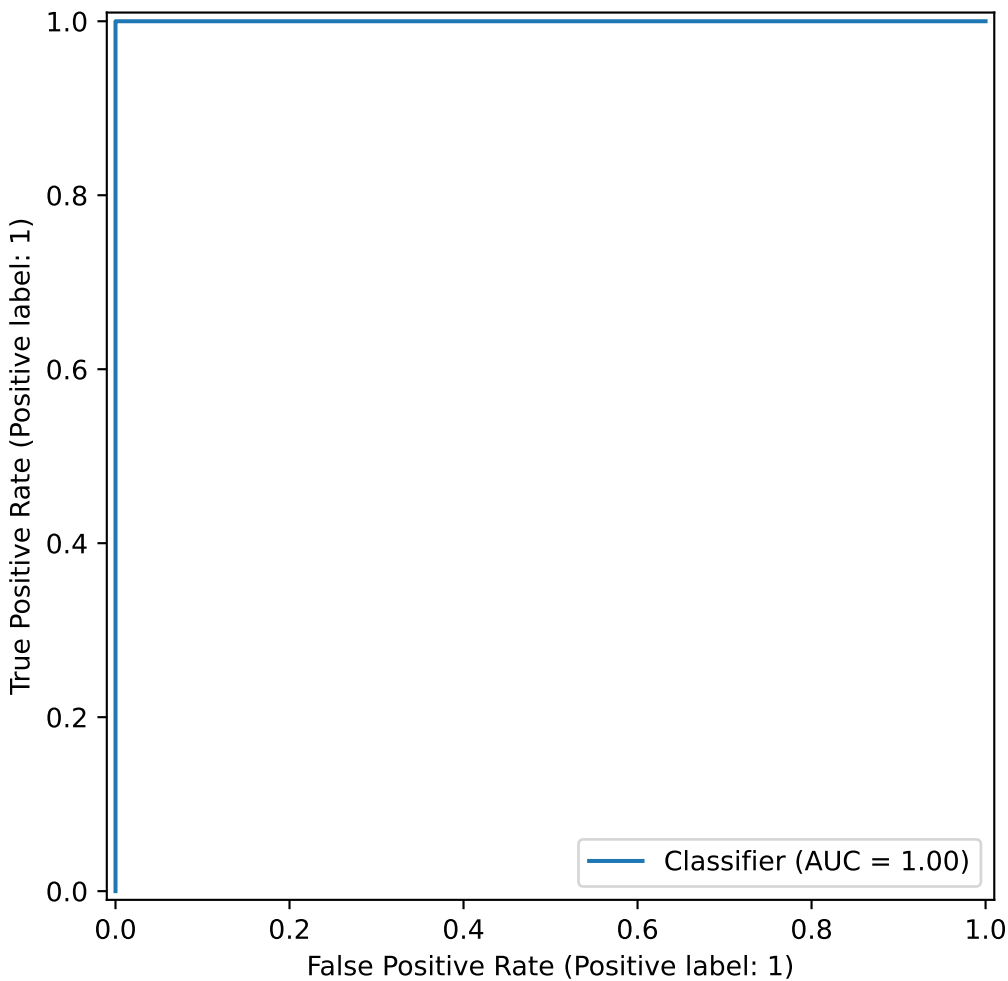
Curva ROC
