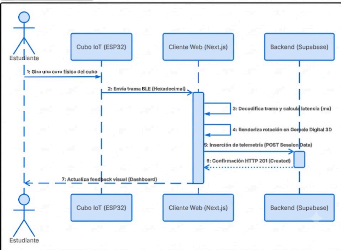
Diagrama de Secuencia: Giro de Cubo IoT
