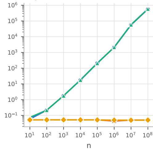
TopBack
