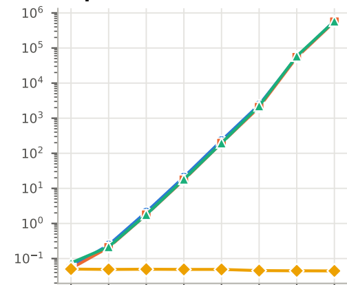
AddAfter
