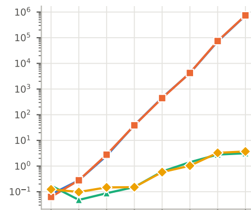
Empty
