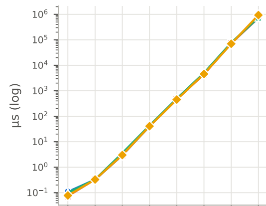
TopFront
