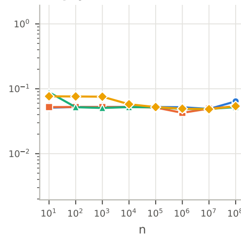
Empty
