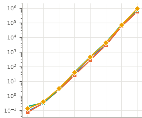
TopBack
