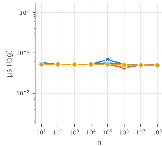
TopFront
