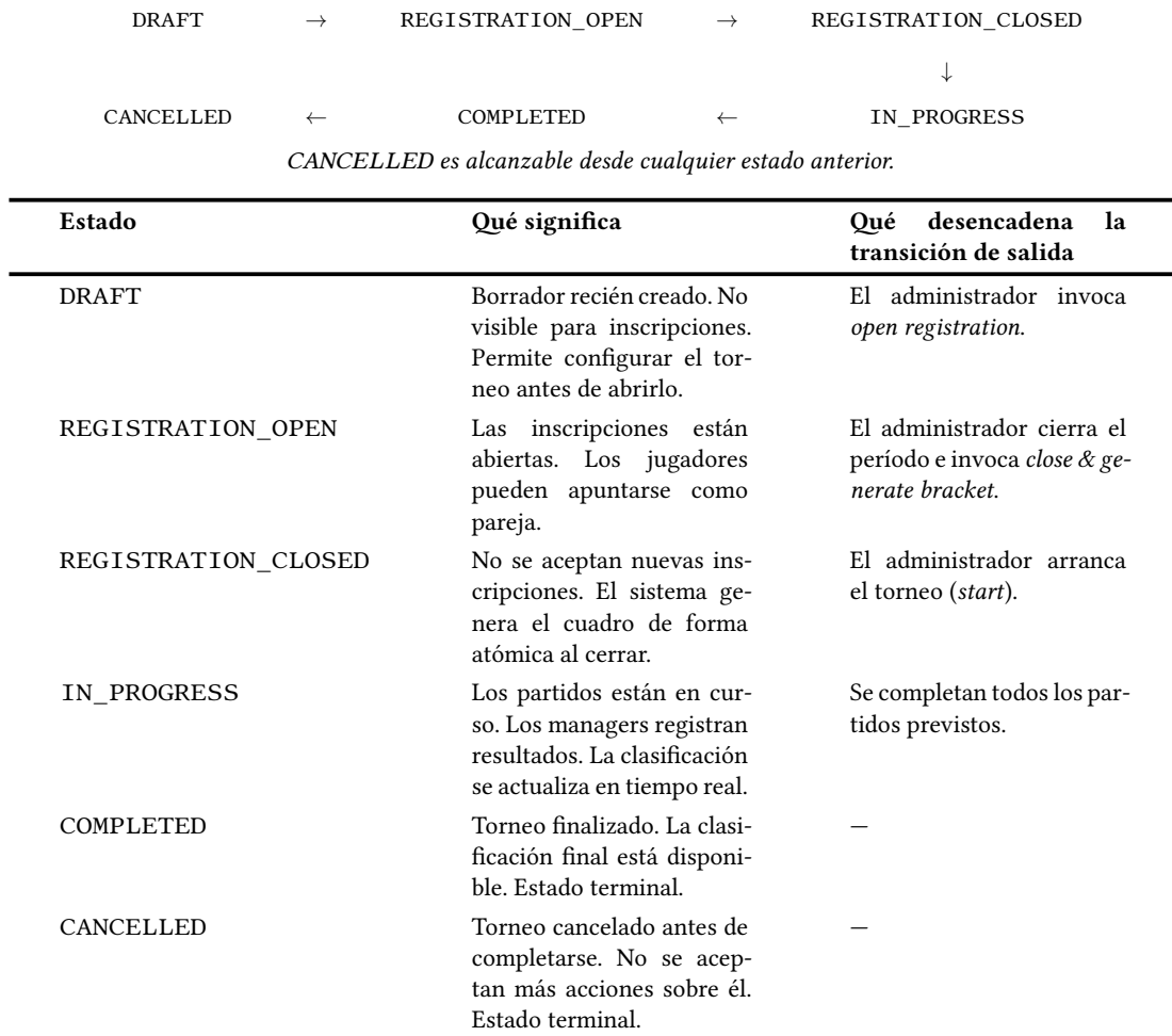
Figura 3.1: Ciclo de vida de un torneo: estados, descripción y transiciones.
