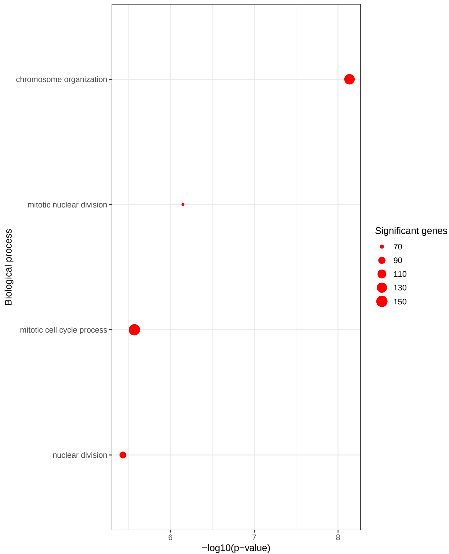
BP_liver_spleen_age_dotplot
